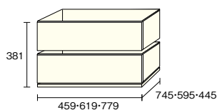
●寸法図 (mm)
