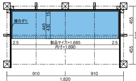
●平面図 (mm) 6尺タイプの場合
