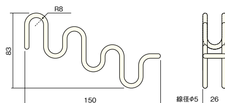
③寸法図 (mm)
