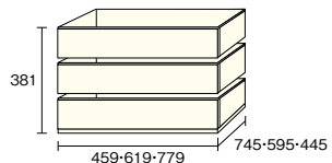
●寸法図 (mm)
