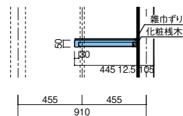
●横断面図 (mm)
