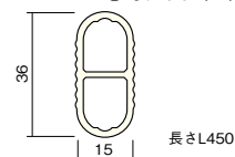
③寸法図 (mm)
