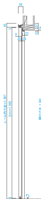
■縦断面図 [レールタイプ]
