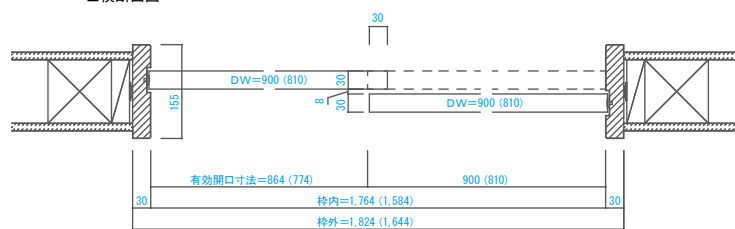
■横断面図
