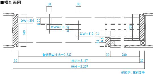
■横断面図
