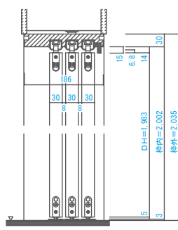
■縦断面図〔床直付けレールタイプ〕
