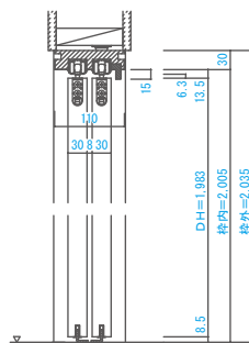
■ 縦断面図
