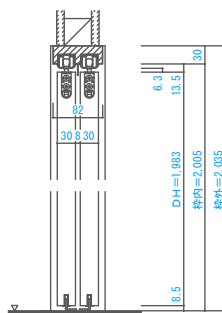
■ 縦断面図
