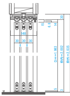
■縦断面図[床直付けレールタイプ]
