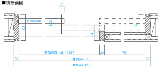
■横断面図
