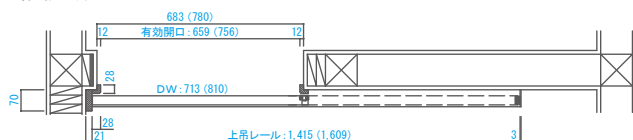
■両入隅・縦枠 納まり図
