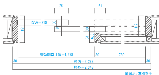
■横断面図
