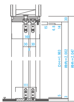
■縦断面図[レールタイプ]
