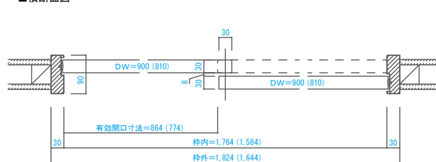
■横断面図
