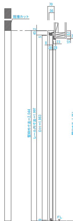
■縦断面図 [レール+縦枠タイプ]
