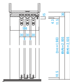
■縦断面図
