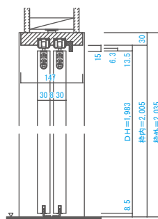
■縦断面図
