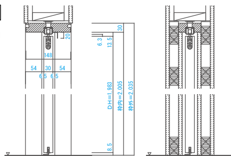
■ 縦断面図
