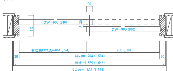
■横断面図
