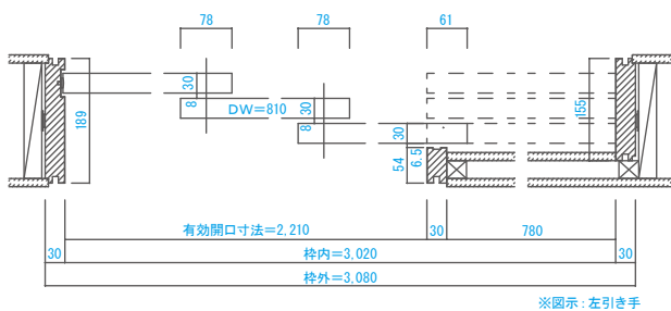
■横断面図
