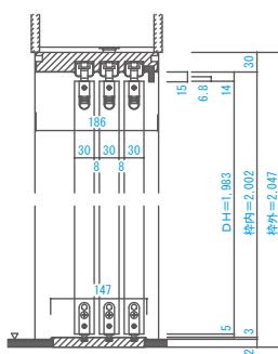
■縦断面図[レールタイプ]
