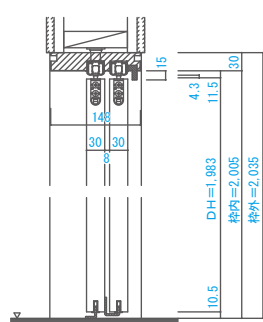
■縦断面図
