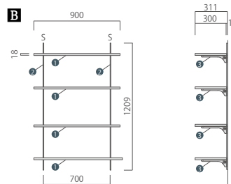
FN-005 B フツウノブラケットプラン
