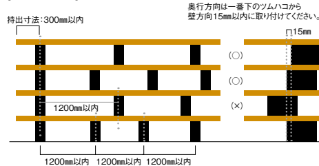
【壁付け仕様の場合】
