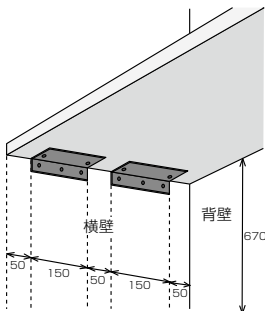
横壁側のL型アンクル取り付け位置
