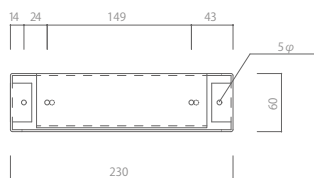
〈共通〉上面図
