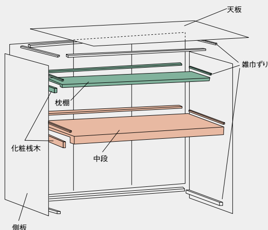
中段・枕棚・パイプハンガーの組み合わせ
