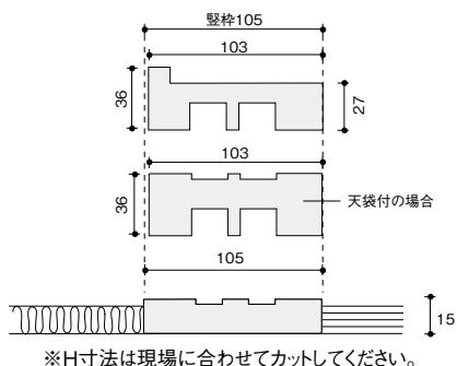
敷居寸法図
