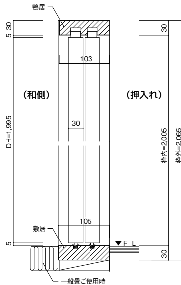
一般畳で使用時(バリアフリー対応)敷居厚30mmタイプ
