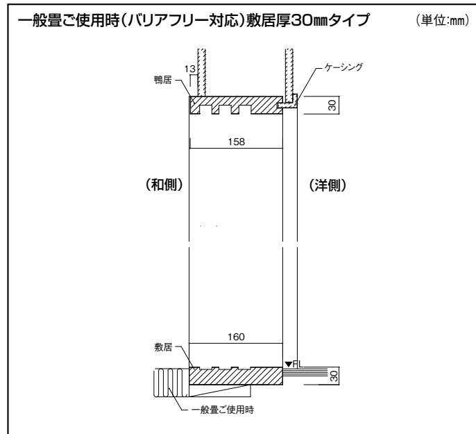
縦断面図
