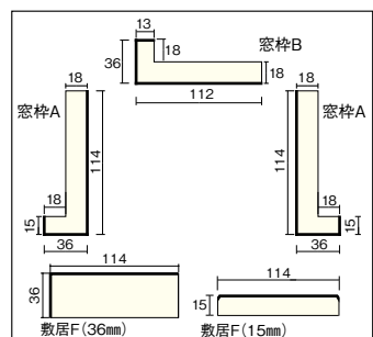
●正寸プレカット対応寸法図(mm)
