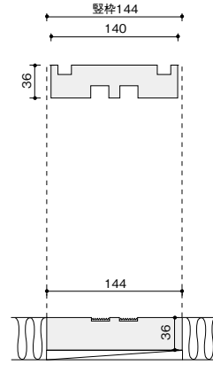
鴨居拡大図
