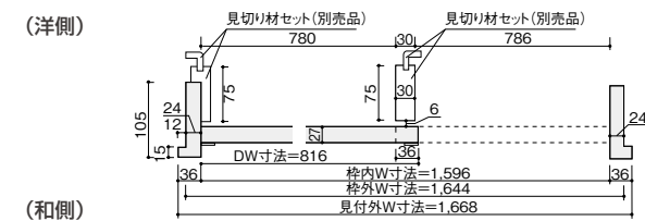
片引き戸(和側引き込み) (単位: mm)
