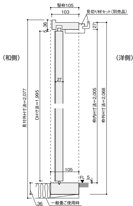
一般置ご使用時(バリアフリー対応)敷居厚36mmタイプ (単位: mm)
