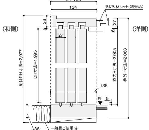
緊栓136 (単位: mm)
