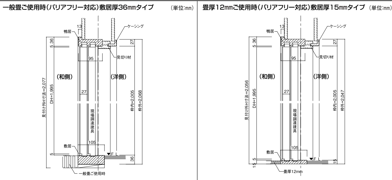
縦断面図
