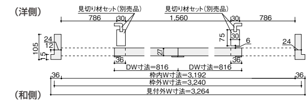
引き分け戸(和側引き込み) (単位: mm)
