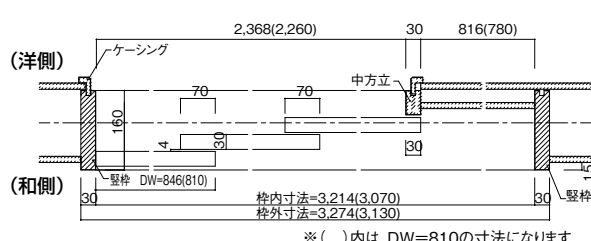
3枚引き込み戸(和側引き込み)
