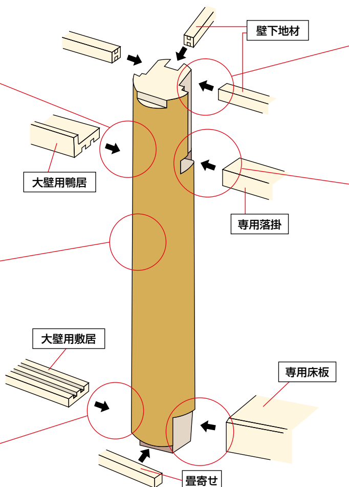
壁下地材との取り合い
