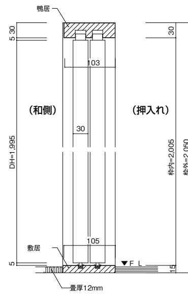
畳厚12mmで使用時(バリアフリー対応)敷居厚15mmタイプ (単位:mm)
