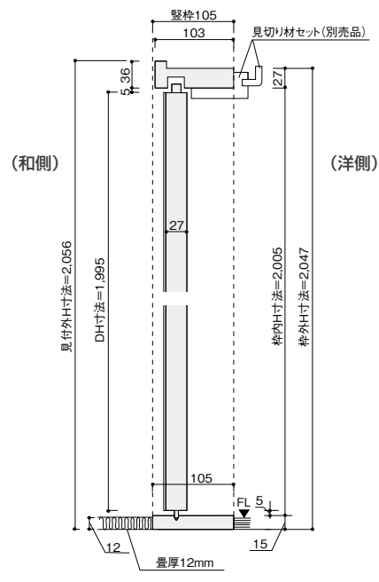
量厚12mmご使用時(バリアフリー対応)敷居厚15mmタイプ (単位: mm)
