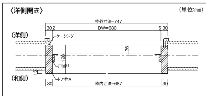
横断面図
