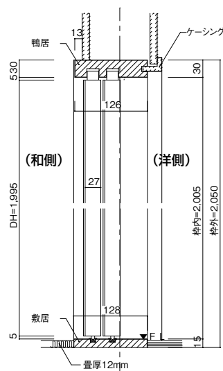
畳厚12mmご使用時(バリアフリー対応)敷居厚15mmタイプ (単位:mm)
