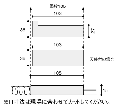
敷居寸法図
