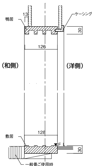
一般畳ご使用時(バリアフリー対応)敷居厚30mmタイプ
