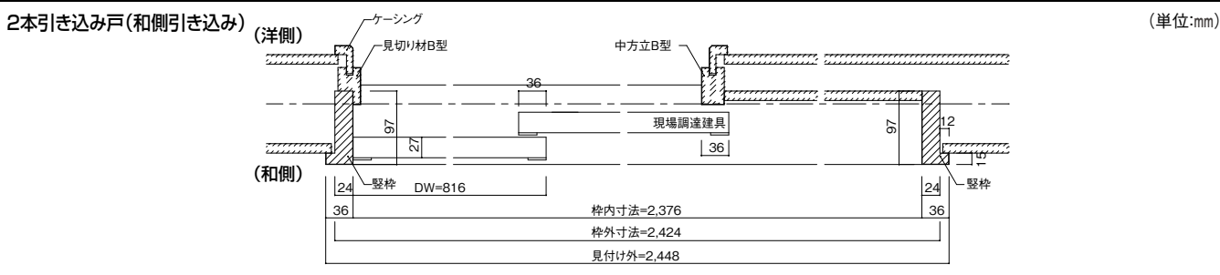
横断面図
