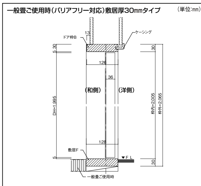
縦断面図
