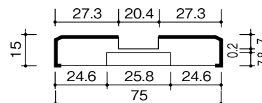
直置き敷居詳細図
