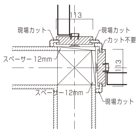
ドアとドアの入隅取り合い
