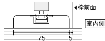
直置き敷居詳細図
