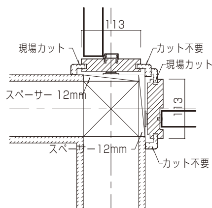
ドアと引戸の入隅取り合い
