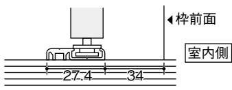
床直付けレール詳細図
