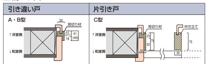
■納まり図
