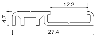
床直付けレール詳細図
