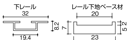
埋め込みレール詳細図
