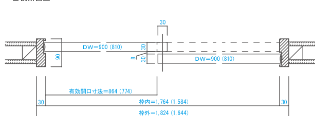
■横断面図
