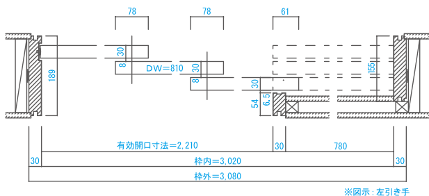
■横断面図
