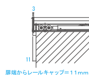
■扉を閉じた時
