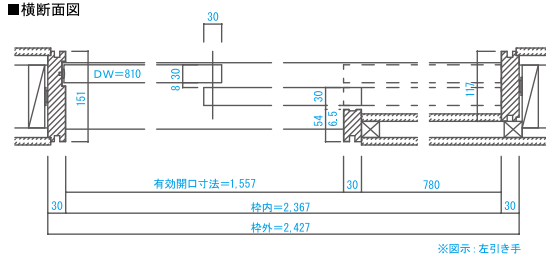
■横断面図
