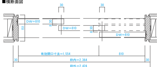
■横断面図
