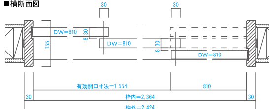
■横断面図
