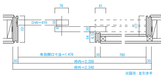
■横断面図
