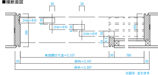
■横断面図
