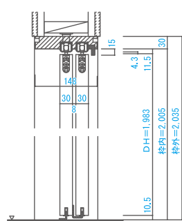
■縦断面図
