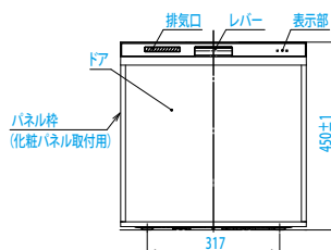
【正面図】
