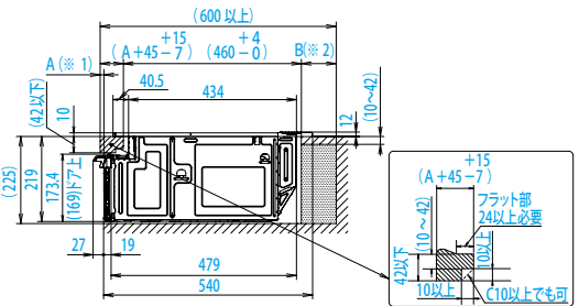
【側面図】
