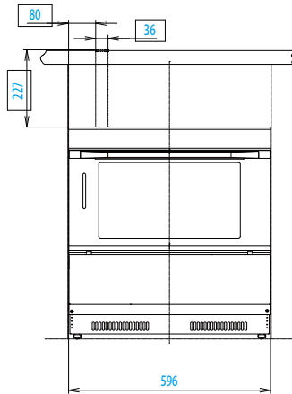
【正面図】
