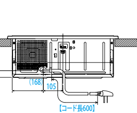
【背面図】
