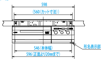
【正面図】
