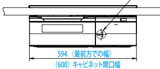
【正面図】
