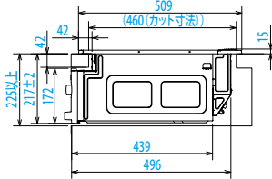
【側面図】
