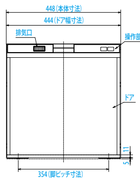
【正面図】
