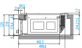
【側面図】
