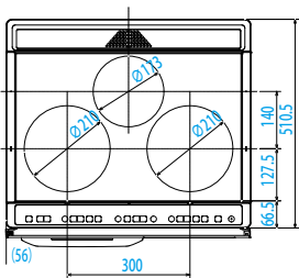
【上面図】
