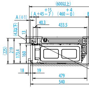
【側面図】
