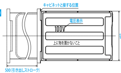
【上面図】
