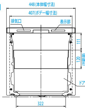
【正面図】
