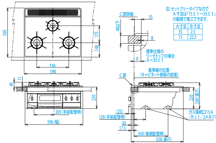
〈設置・配管施工例図(手前側配管時)〉
