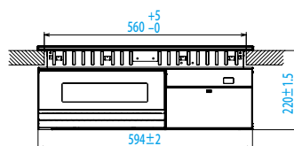
【正面図】
