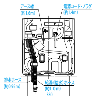
【背面図】
