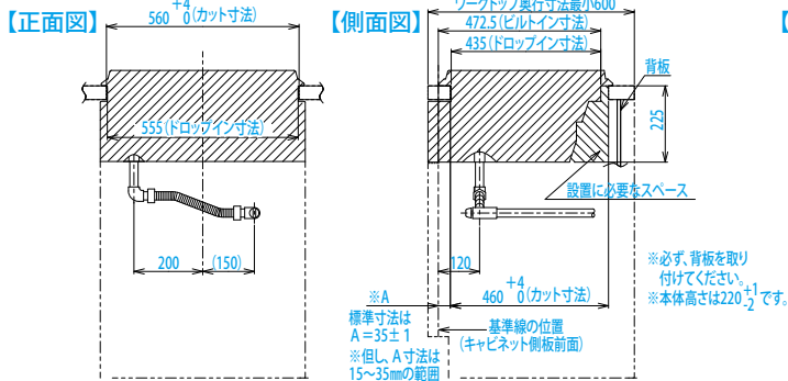
〈設置・配管施工例図(手前側配管時)〉
