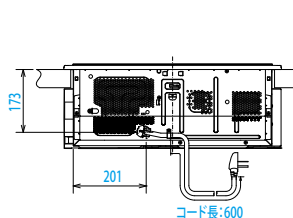
【背面図】
