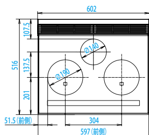
【平面図】
