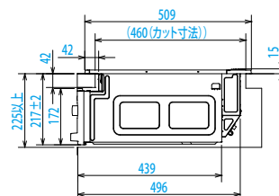
【側面図】
