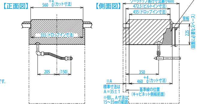
〈設置・配管施工例図(奥側配管時)〉
