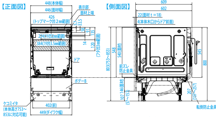
【背面図】
