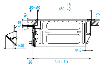
【側面図】 【パネル開閉時】
