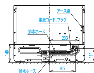
【背面図】
