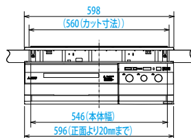
【正面図】
