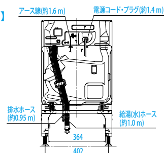
【背面図】
