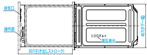
【正面図】
