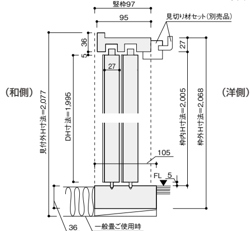
一般量ご使用時(バリアフリー対応)敷居厚36mmタイプ
