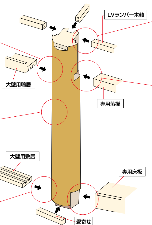
LVランバー木軸との取り合い
