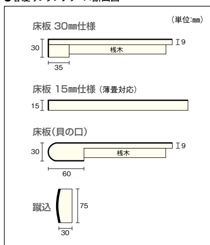
●春慶ウレタンシリーズ断面図
