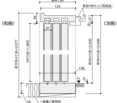
一般量ご使用時(バリアフリー対応)敷居厚36mmタイプ
