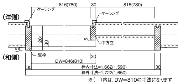
片引き戸(和側引き込み)
