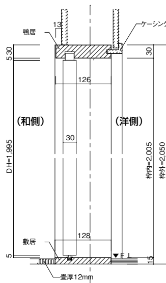
畳厚12mmご使用時(バリアフリー対応)敷居厚15mmタイプ
