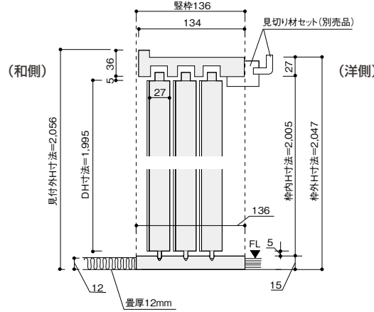
一般量ご使用時(バリアフリー対応)敷居厚36mmタイプ
