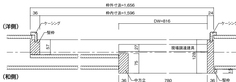
片引き戸(洋側引き込み)
