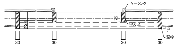
引き分け戸(和側引き込み)
