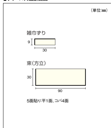
●シリーズ共通断面図
