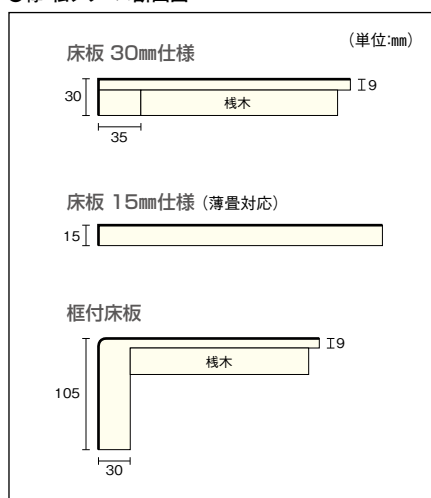
●樺・松シリーズ断面図
