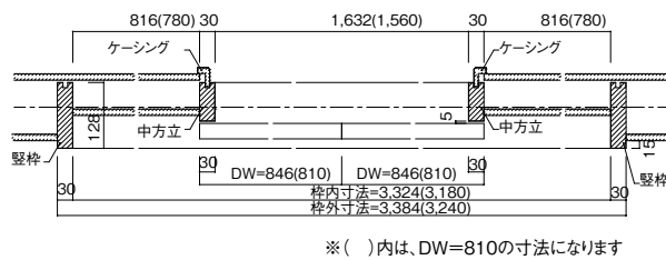
引き分け戸(和側引き込み)
