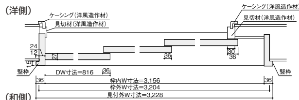
3枚引き込み戸(和側引き込み)
