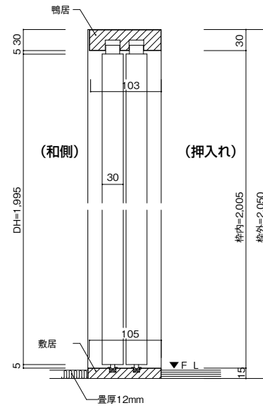
畳厚12mmご使用時(バリアフリー対応)敷居厚15mmタイプ (単位:mm)
