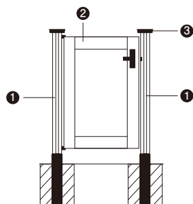
GL埋込み用(木製フェンス扉)部材 H1,100タイプ
