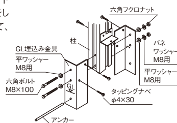
下棧固定金具
