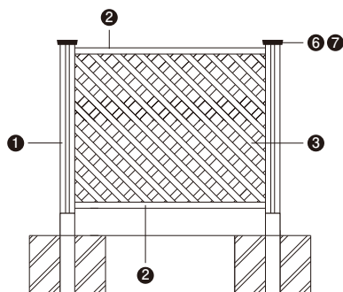
ラチスタイプ H2,200
