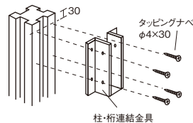
柱・桁連結金具
