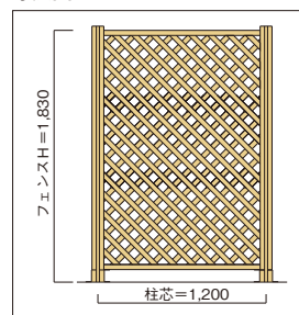
寸法図
