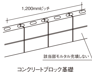
コンクリートブロック基礎
