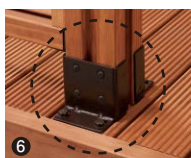
柱固定金具 オリジナルの専用ボルトを ご使用ください。
