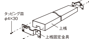
上棧固定金具
