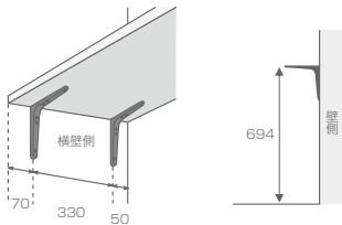
横壁側のカウンターブラケット取り付け位置
