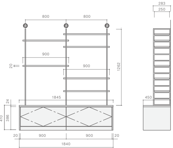
※画像中のTVサイズ…19インチ ●棚板を数枚置けるブラケット
