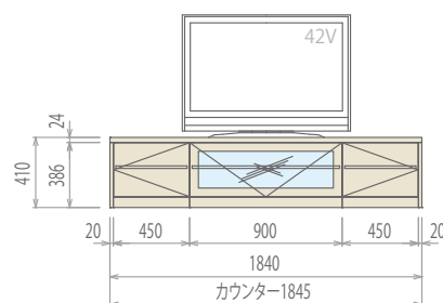
LB-015 W1800 フラップダウン+開き
