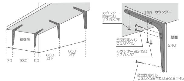
横壁側のカウンターブラケット取り付け位置と間口方向の取り付け位置
