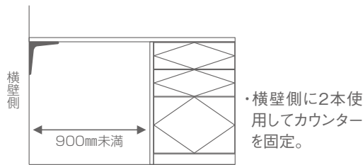
横壁側のカウンターブラケット取り付け位置
