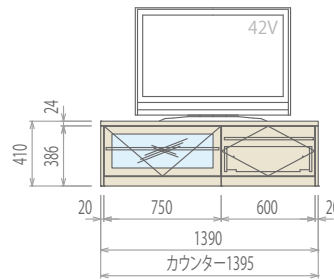
LB-011 W1350 フラップダウン+引出し
