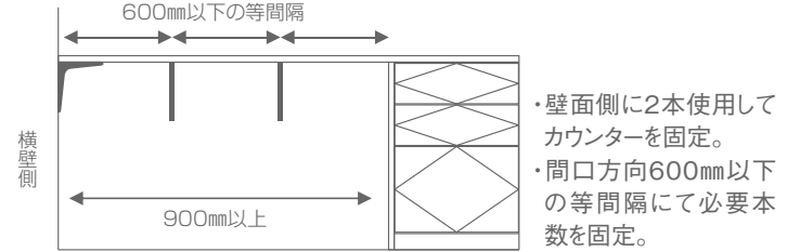
横壁側のカウンターブラケット取り付け位置と間口方向の取り付け位置
