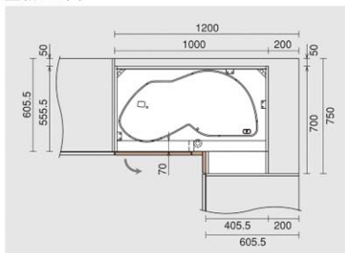
□納まり図
