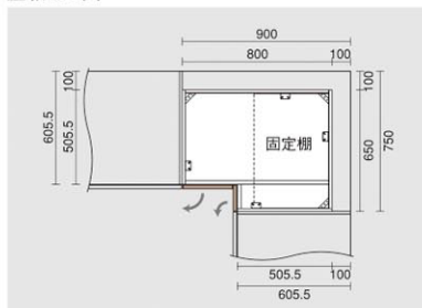
□納まり図
