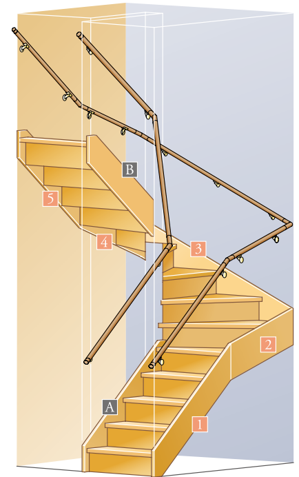
(例)直4段 + 廻り6段 + 直4段
