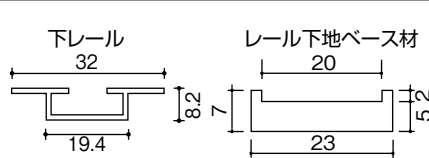
埋め込みレール詳細図
