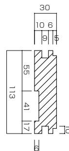
縦枠(開口部側)
