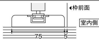
直置き敷居詳細図
