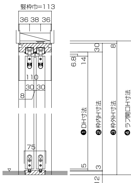
■ 納まり寸法表
