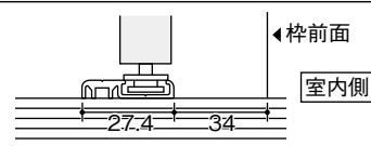
床直付けレール詳細図
