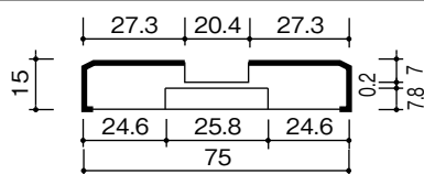
直置き敷居詳細図
