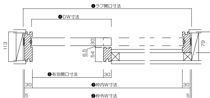
床埋め込み敷居
