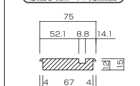
敷居(突板タイプ)加工図
