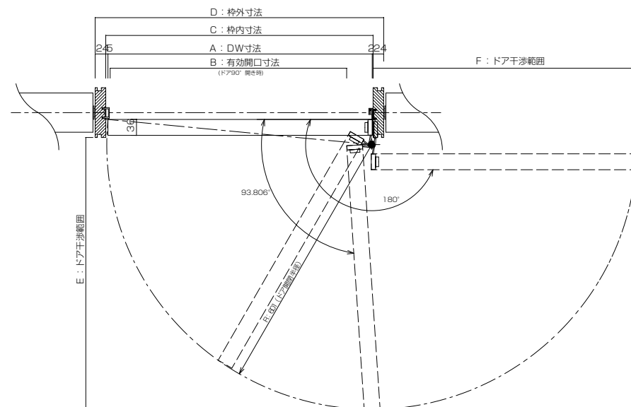
ドアサイズ別の関連寸法表
