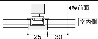
埋め込みレール詳細図
