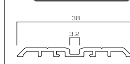
床直付レール図
