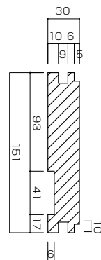
縦枠(開口部側)
