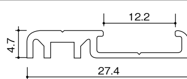
床直付けレール詳細図
