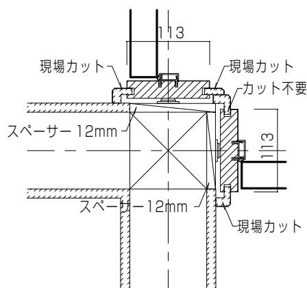
ドアとドアの入隅取り合い
