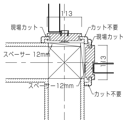
ドアと引戸の入隅取り合い
