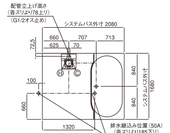
排水・給水給湯位置図
