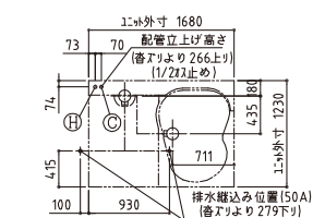
排水・給水給湯位置図
