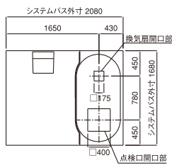
アーチ天井開口位置図
