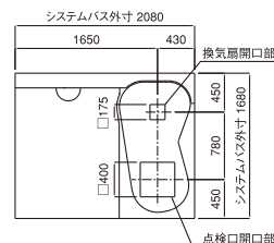
アーチ天井開口位置図
