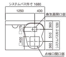
アーチ天井開口位置図
