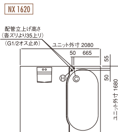
給水給湯位置図
