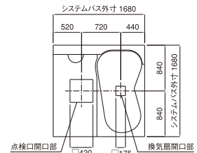
フラット天井開口位置図
