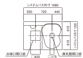
フラット天井開口位置図
