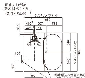
排水・給水給湯位置図
