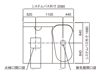
フラット天井開口位置図
