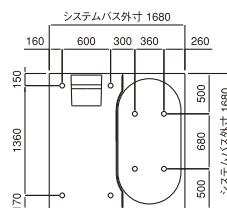
設置脚位置図
