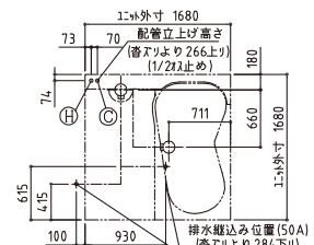
排水・給水給湯位置図
