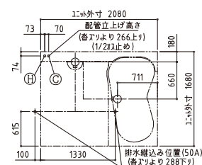
排水・給水給湯位置図
