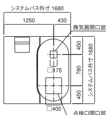
アーチ天井開口位置図
