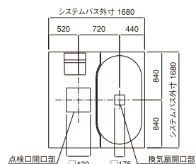
フラット天井開口位置図
