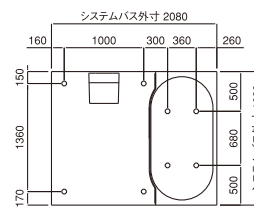
設置脚位置図
