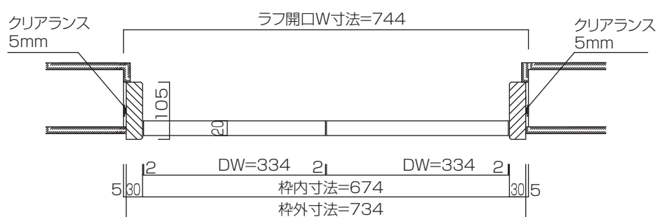
横断面図
