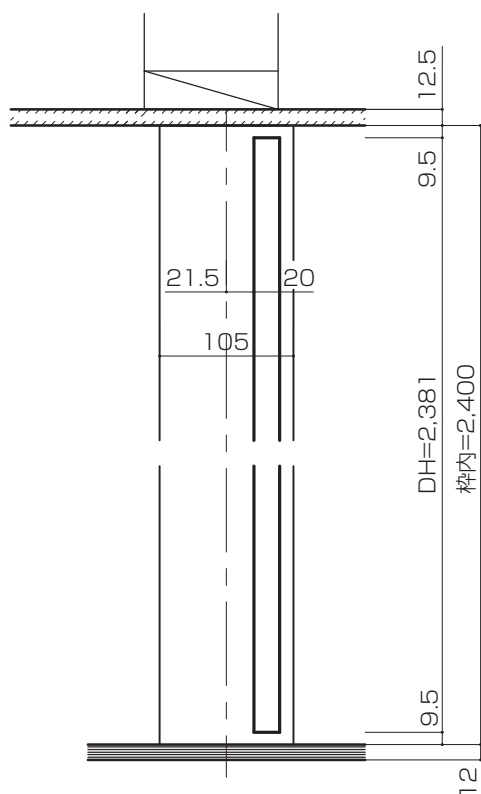
横断面図
