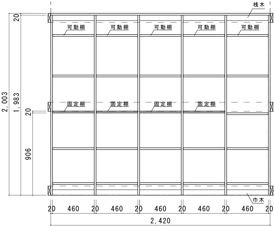
正面展開図
