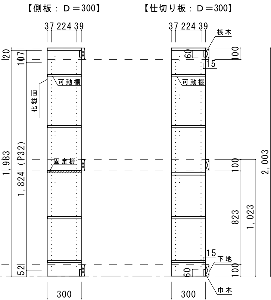
a-a 断面図
