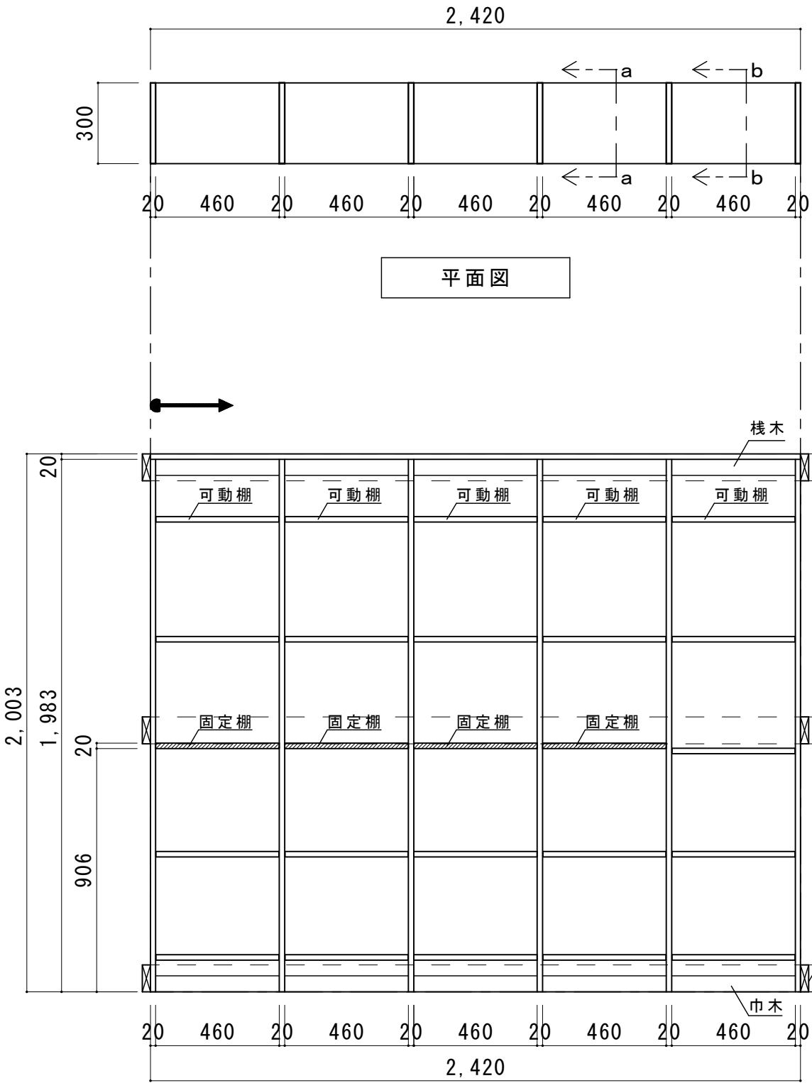
正面展開図
