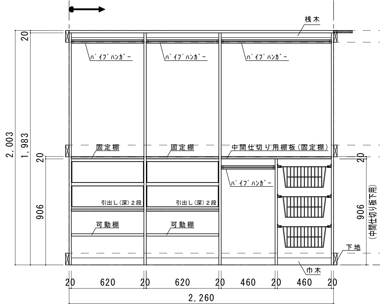
正面展開図
