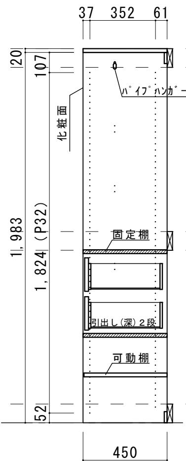
a-a 断面図
