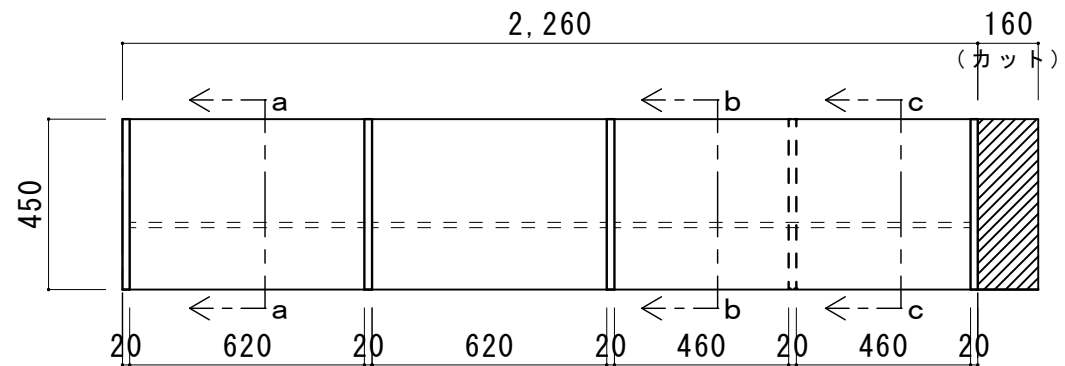
平面図
