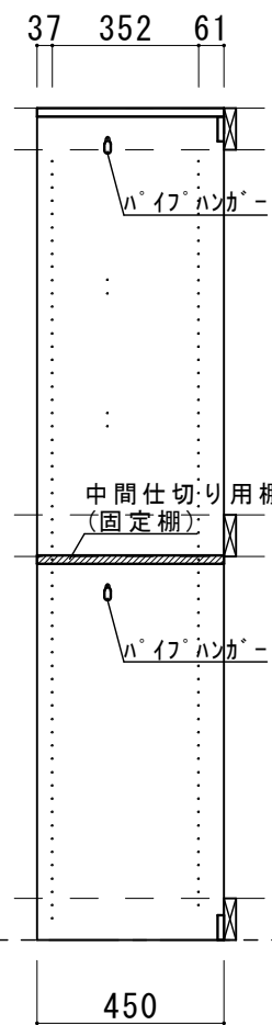
b-b 断面図
