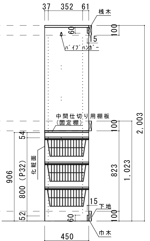
c-c 断面図
