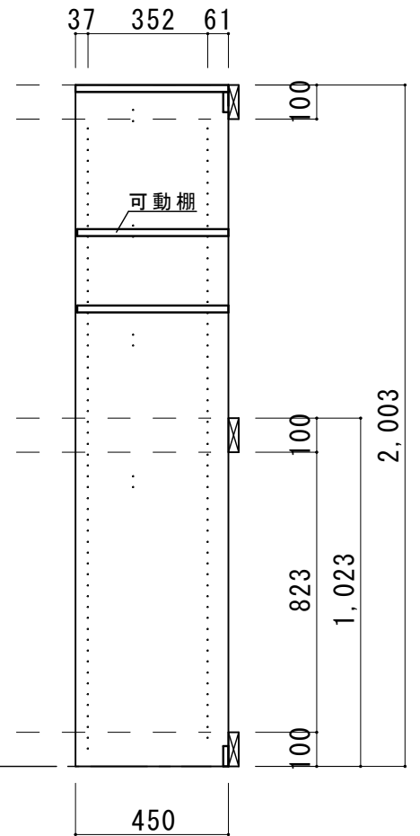
d-d 断面図
