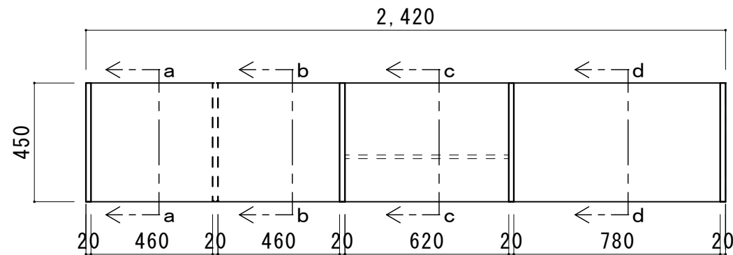
平面図
