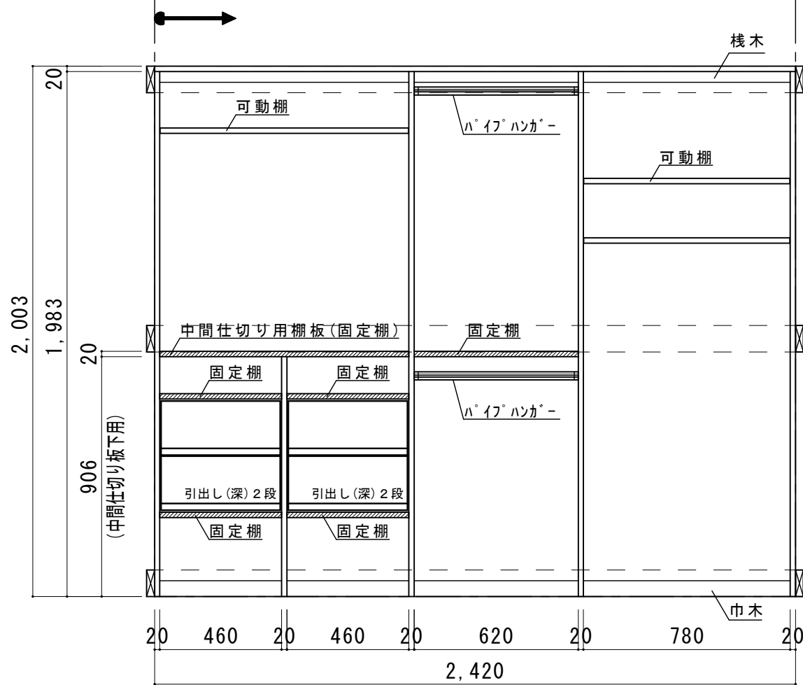
正面展開図
