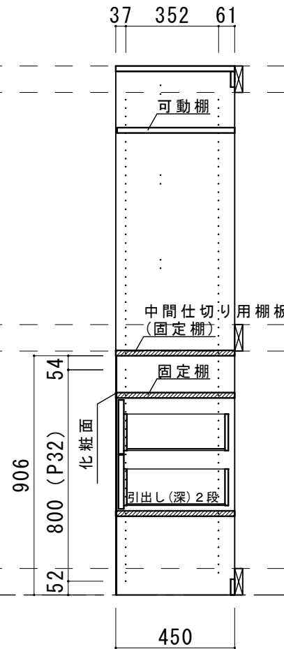
b-b 断面図
