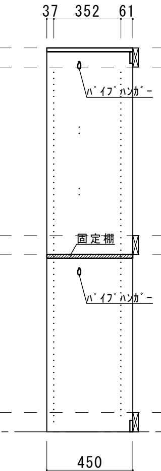
c-c 断面図
