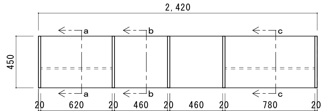
平面図
