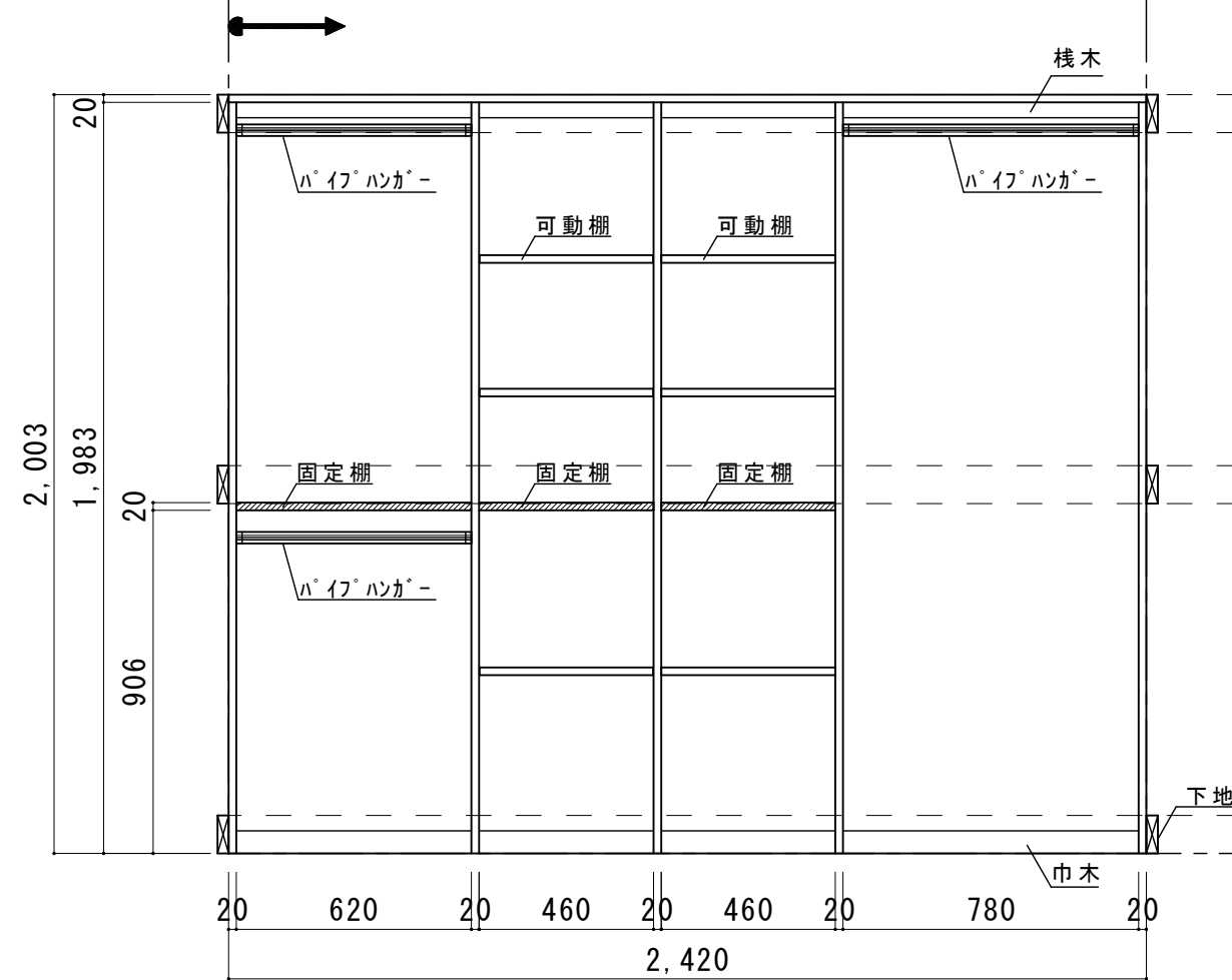
正面展開図
