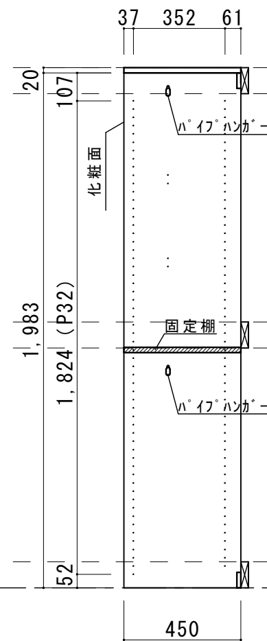
【側板：D=450】
