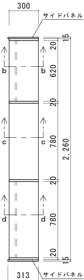
B 面
