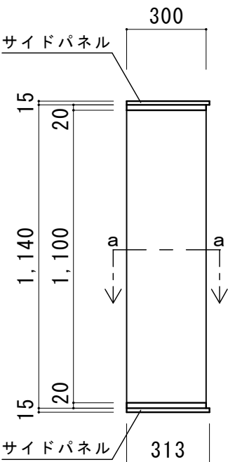
A 面
