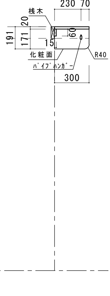
c-c 断面図
