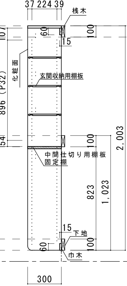
b-b 断面図
