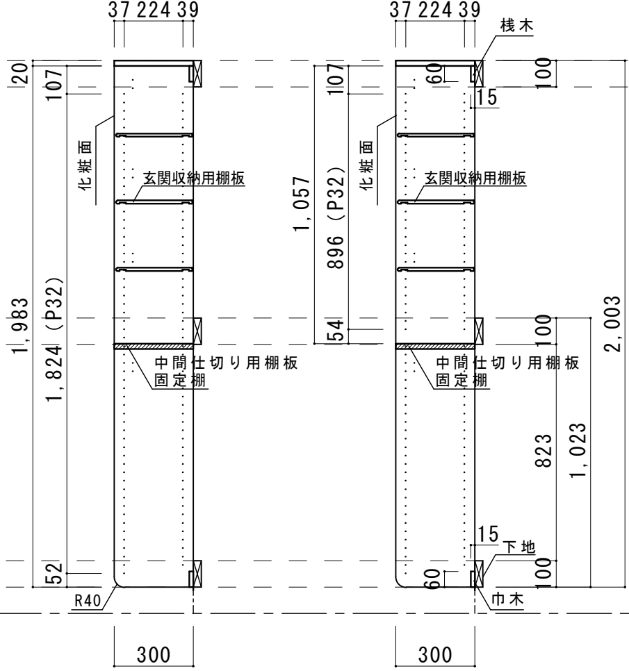
a-a 断面図
