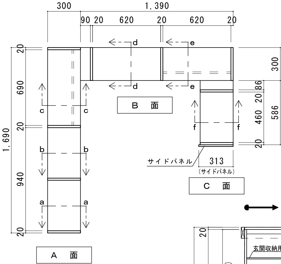
全体平面図
