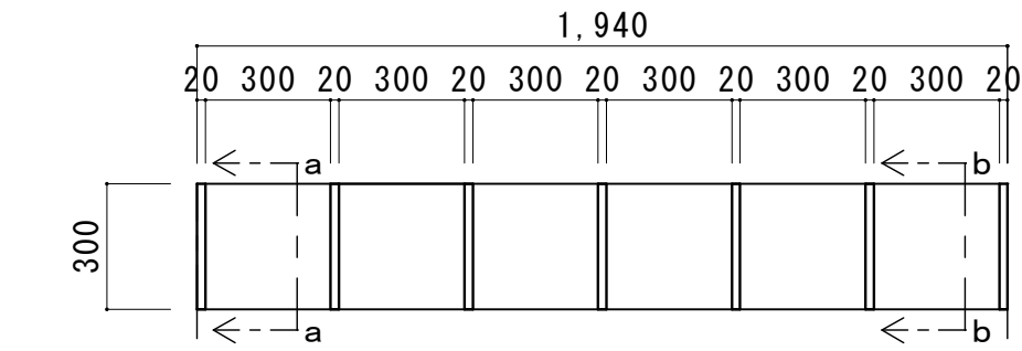
上部平面図
