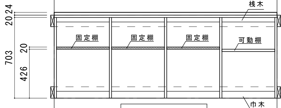
正面展開図
