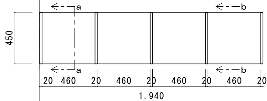
下部平面図
