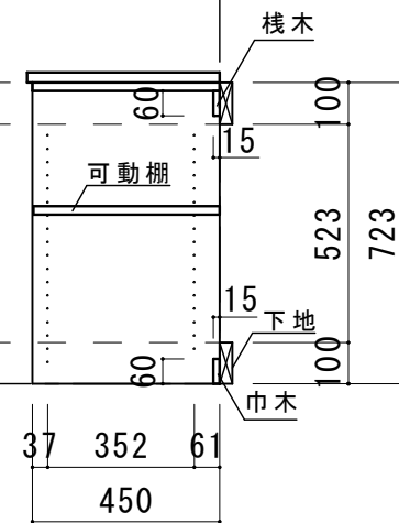
b - b 断面図
