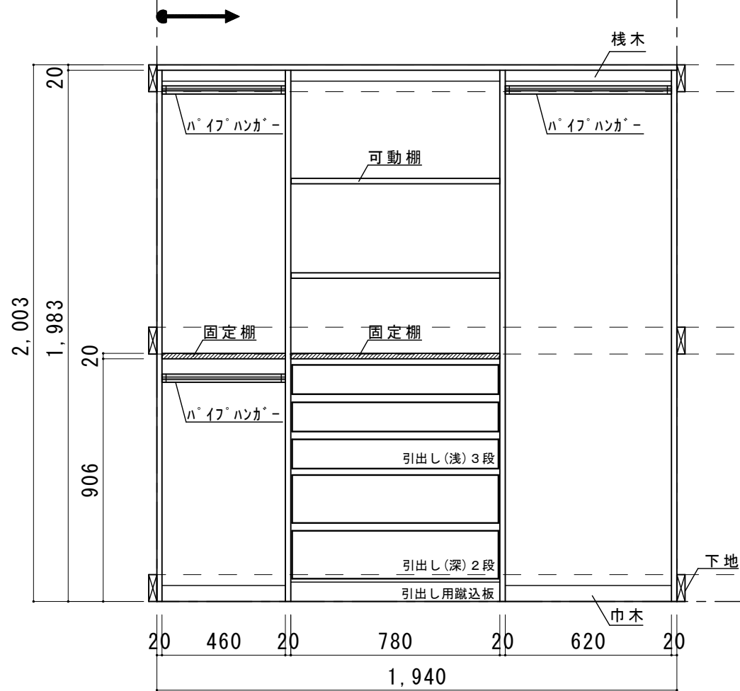
正面展開図
