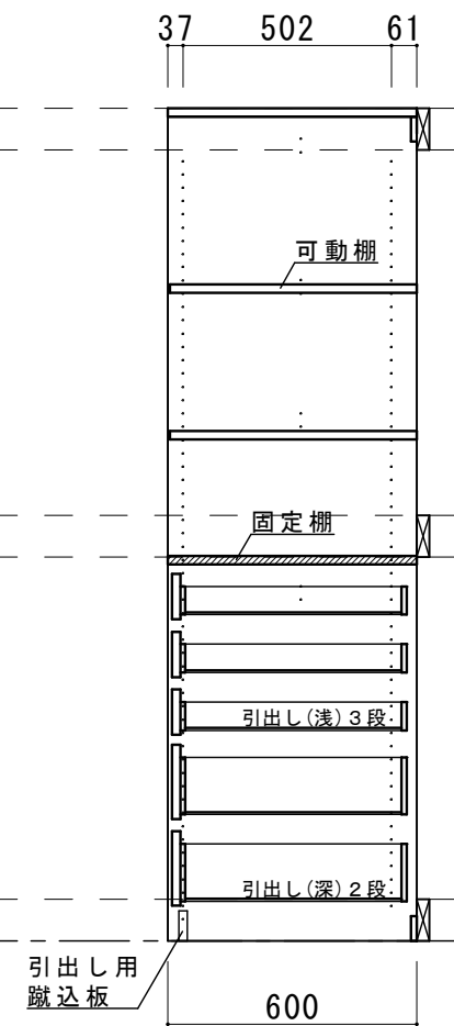
b-b 断面図
