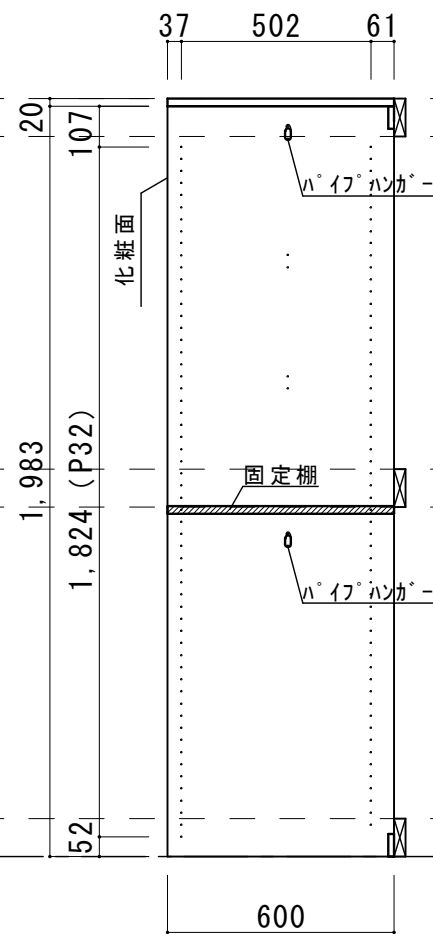
a-a 断面図
