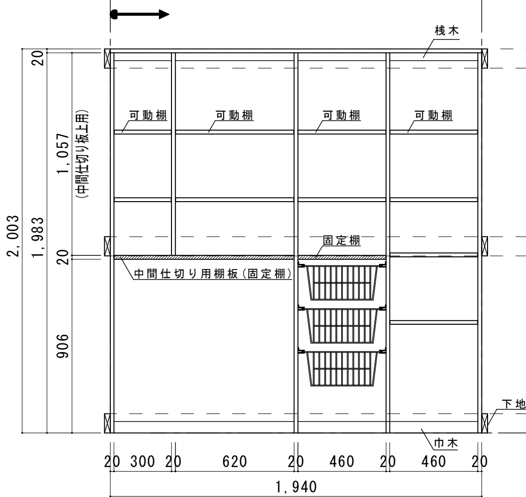
正面展開図
