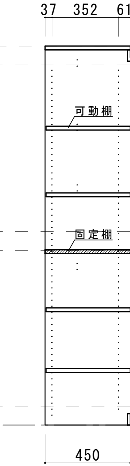
【仕切り板：D=450】
