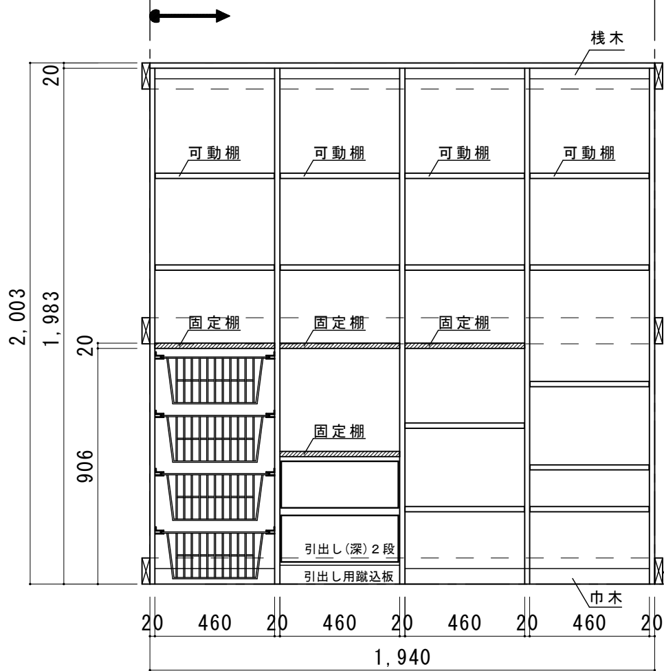
正面展開図
