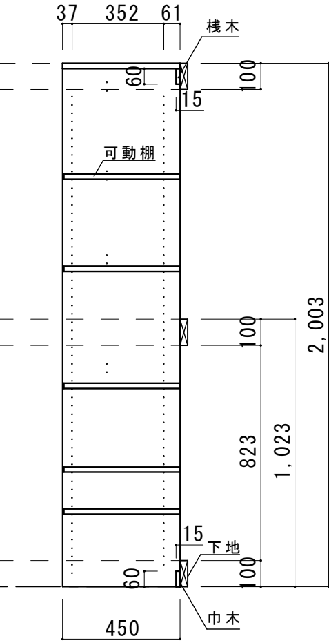
【仕切り板：D=450】
