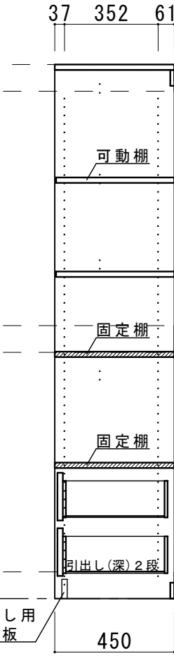
【仕切り板：D=450】
