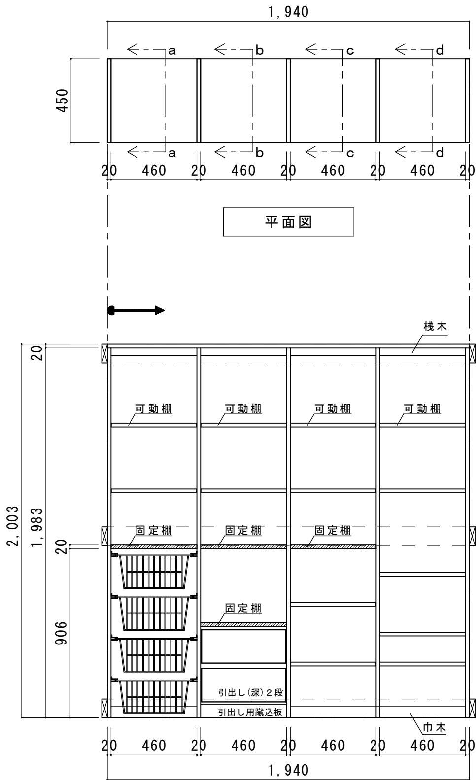
正面展開図
