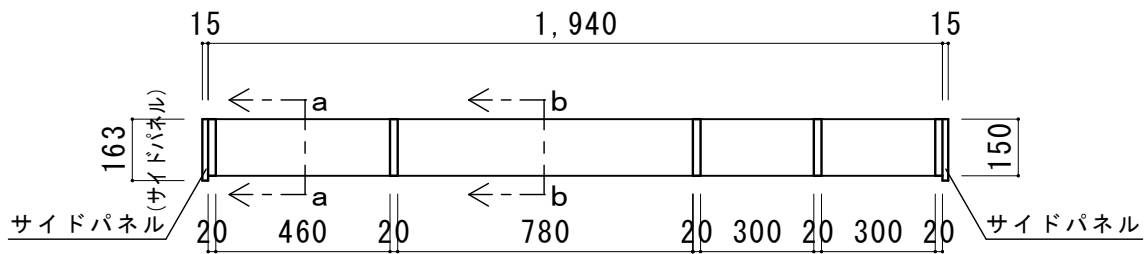
平面図
