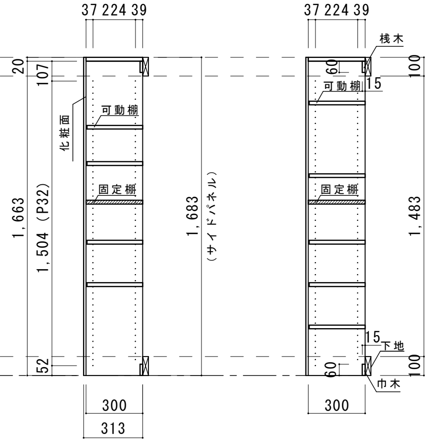
a-a 断面図
