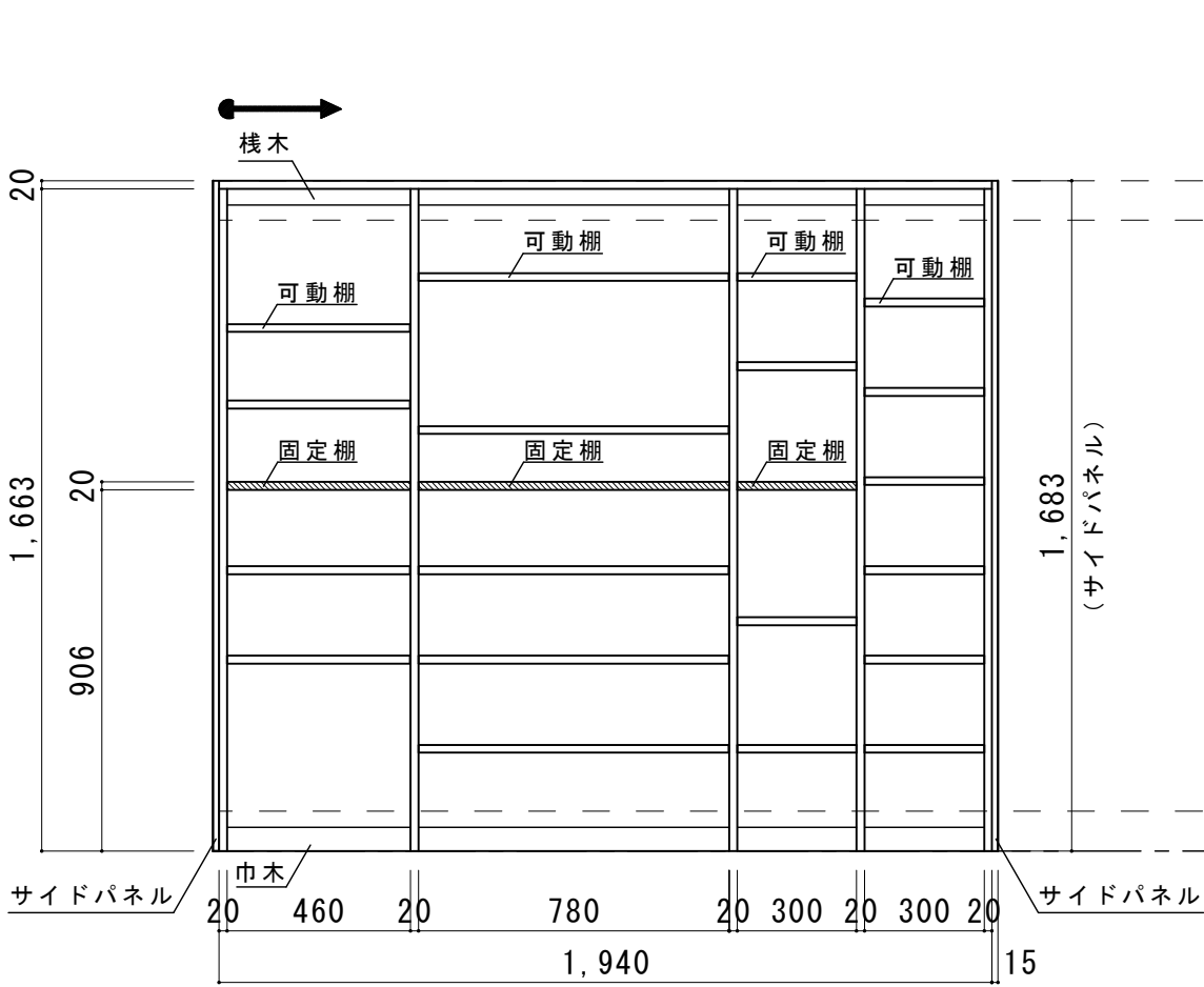
正面展開図
