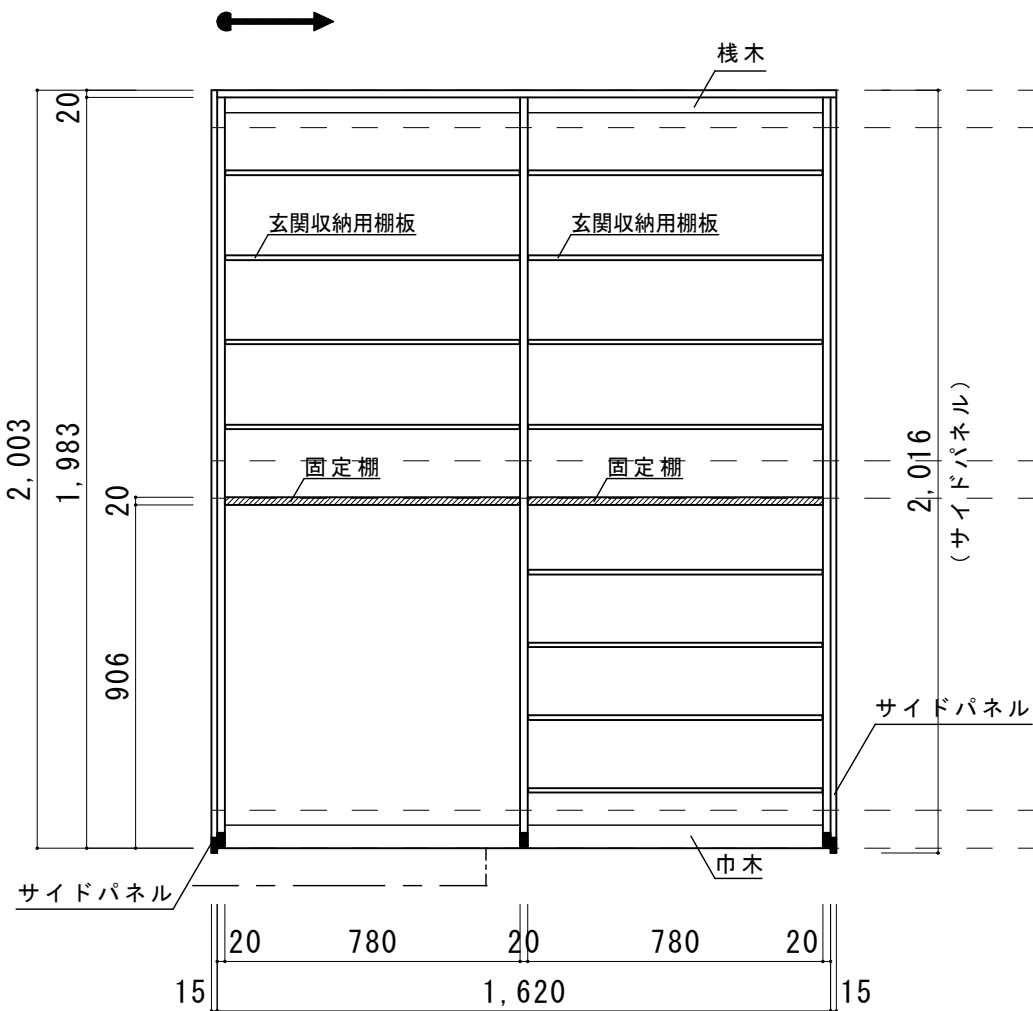
正面展開図
