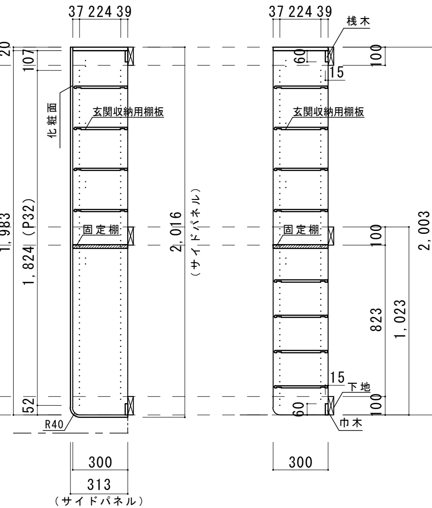
a-a 断面図
