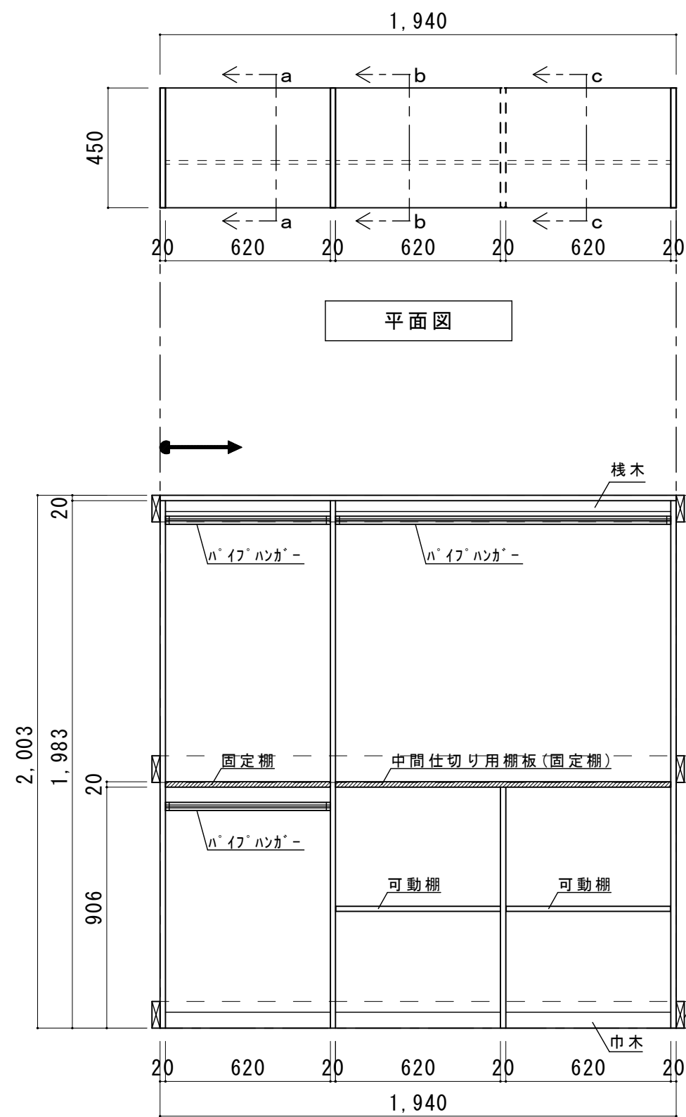
正面展開図
