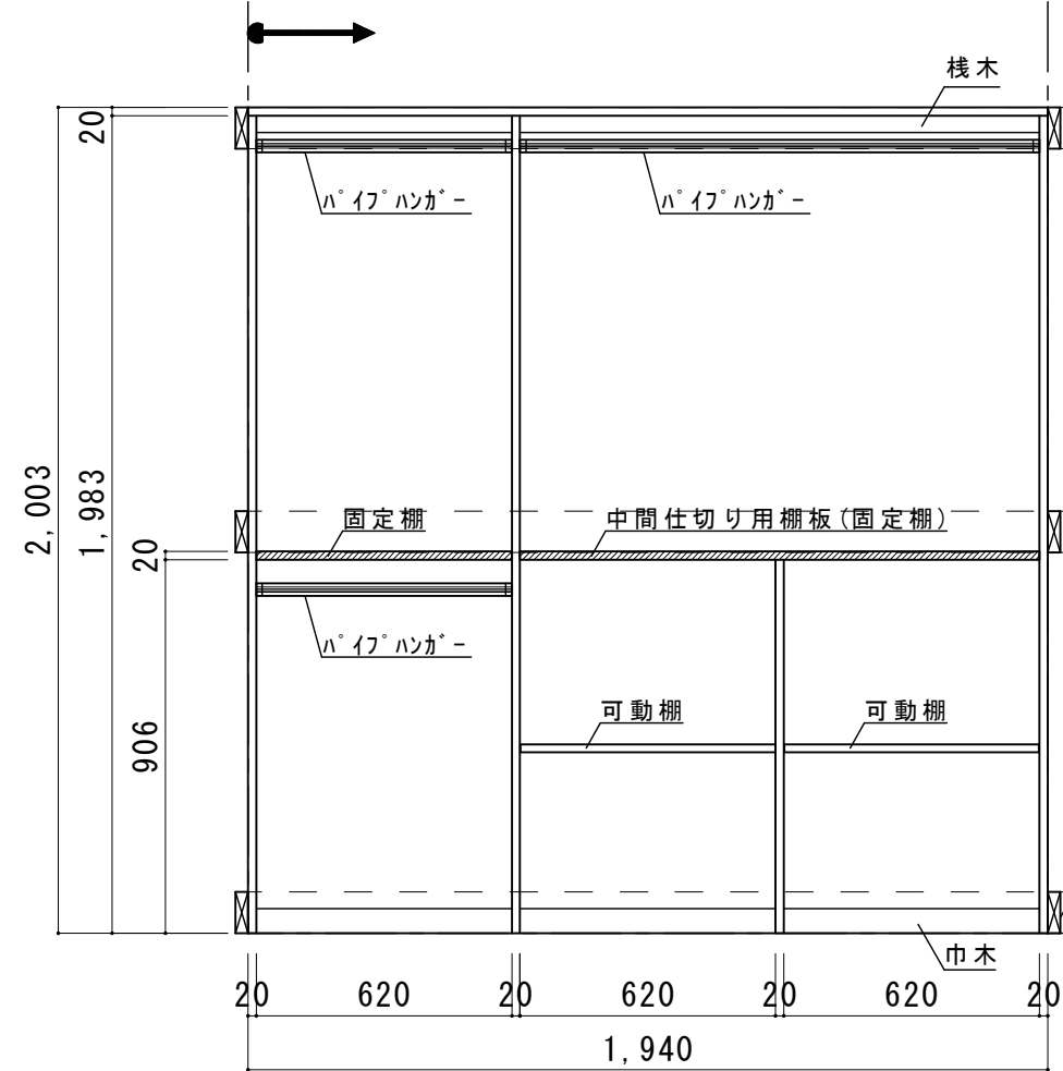
正面展開図
