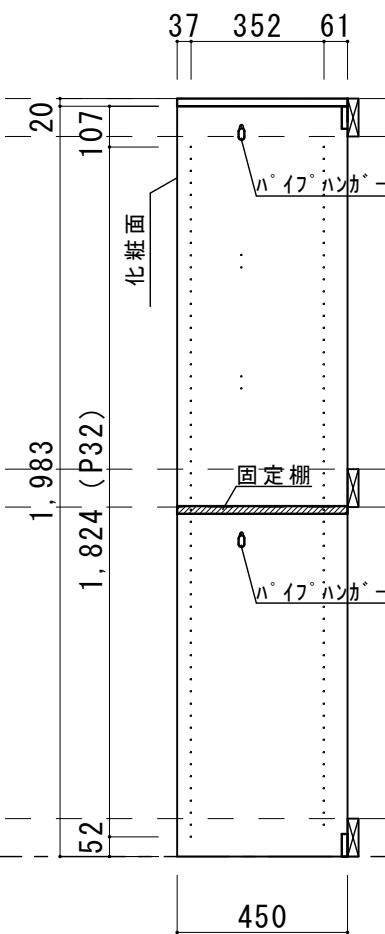
【側板 : D=450】
