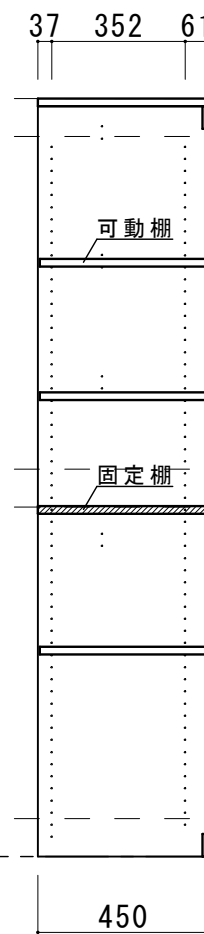
b - b 断面図
