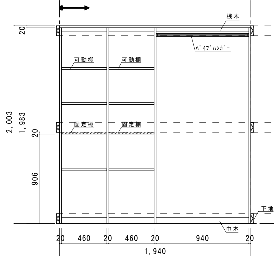
正面展開図
