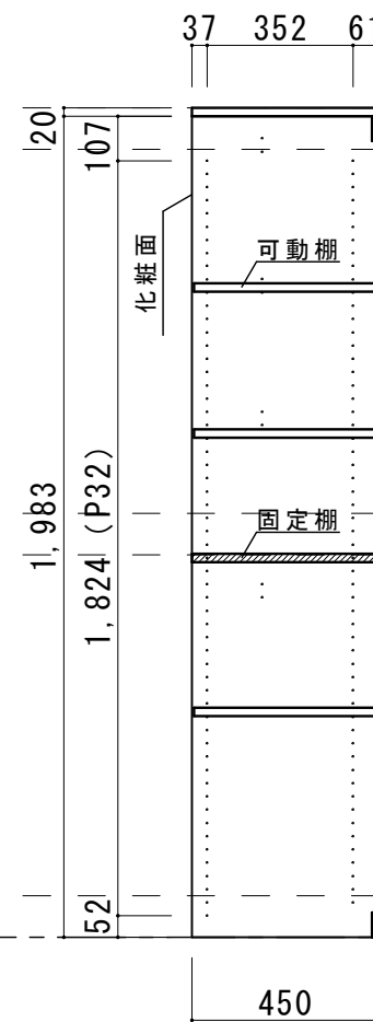
a - a 断面図
