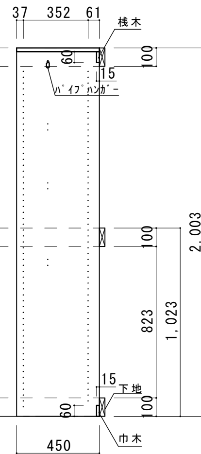
c - c 断面図
