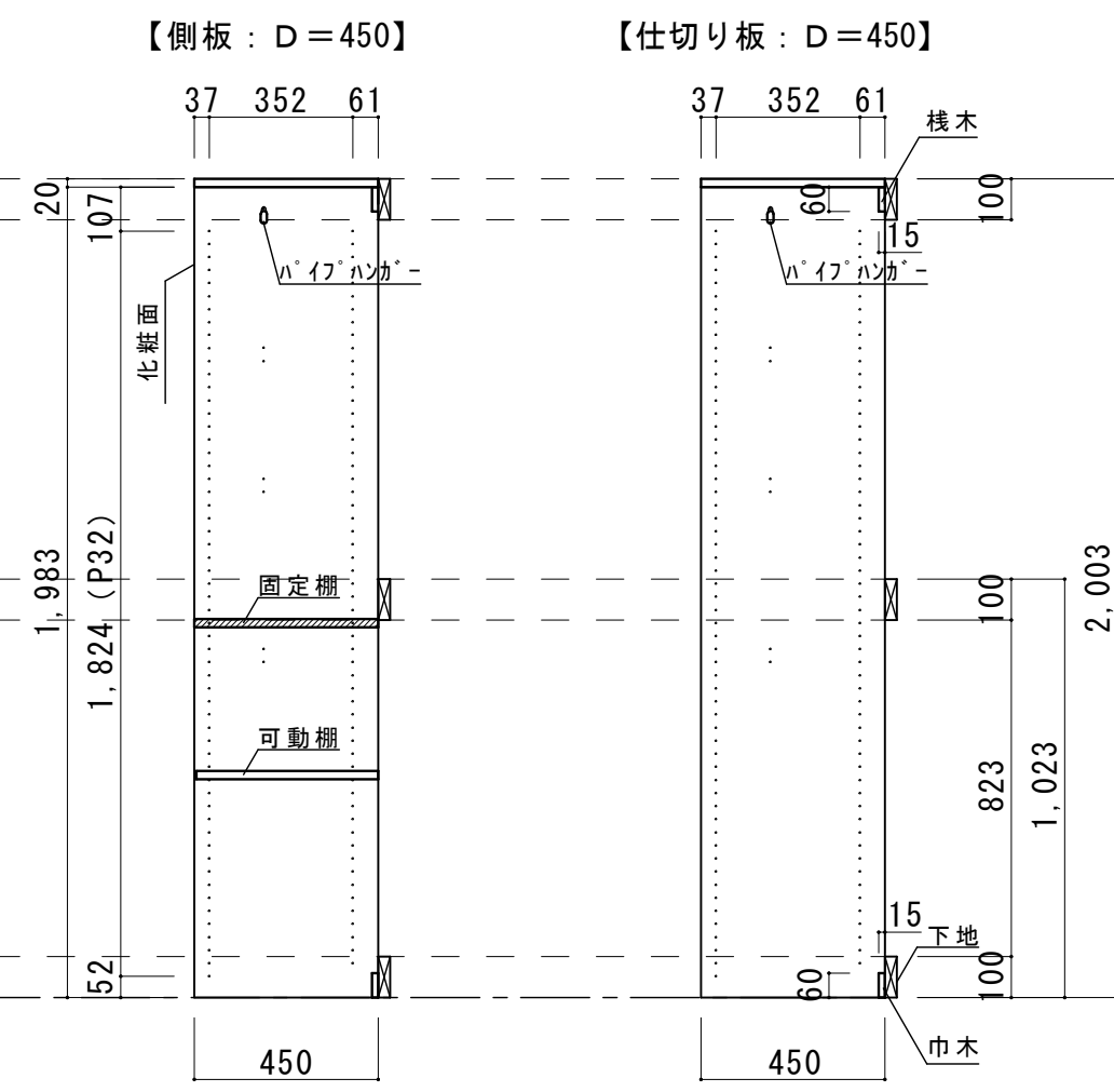
a - a 断面図
