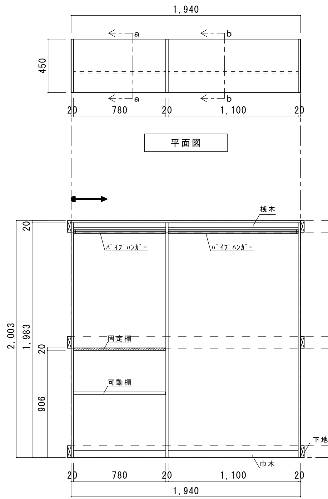
正面展開図
