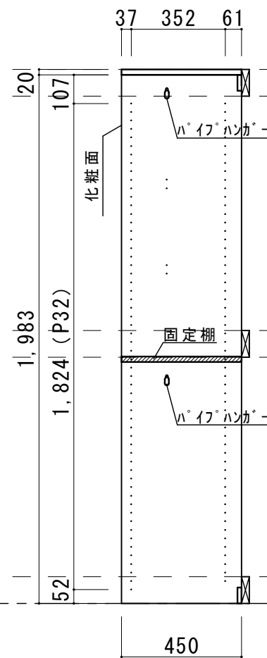
a-a 断面図
