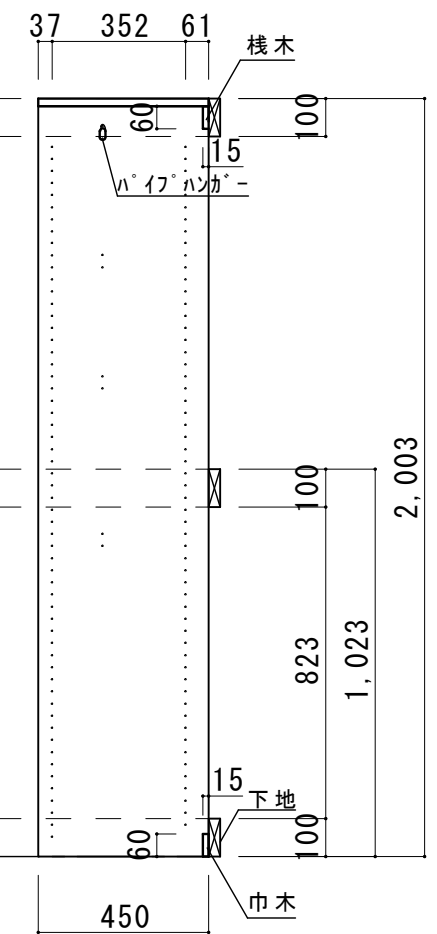
c-c 断面図
