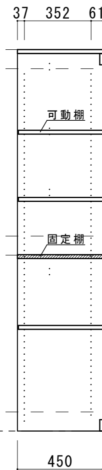
b-b 断面図
