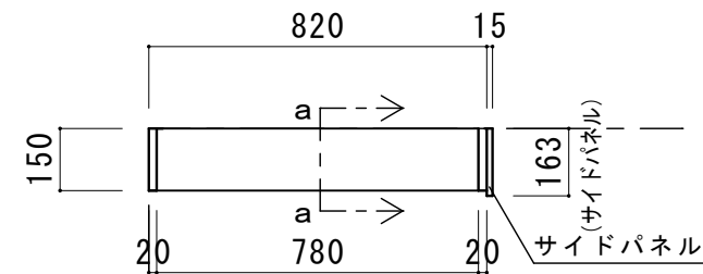
上部平面図
