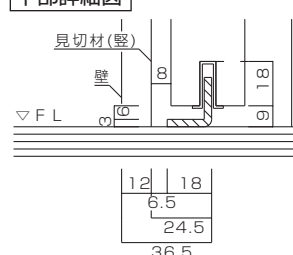
下部詳細図
