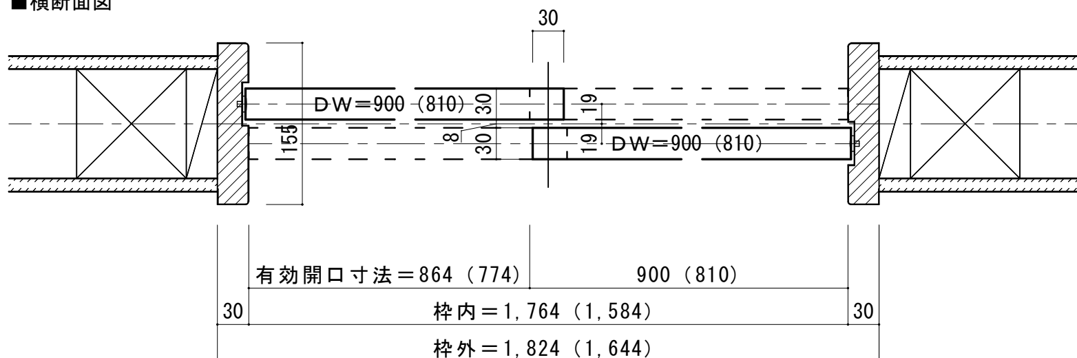
■横断面図
