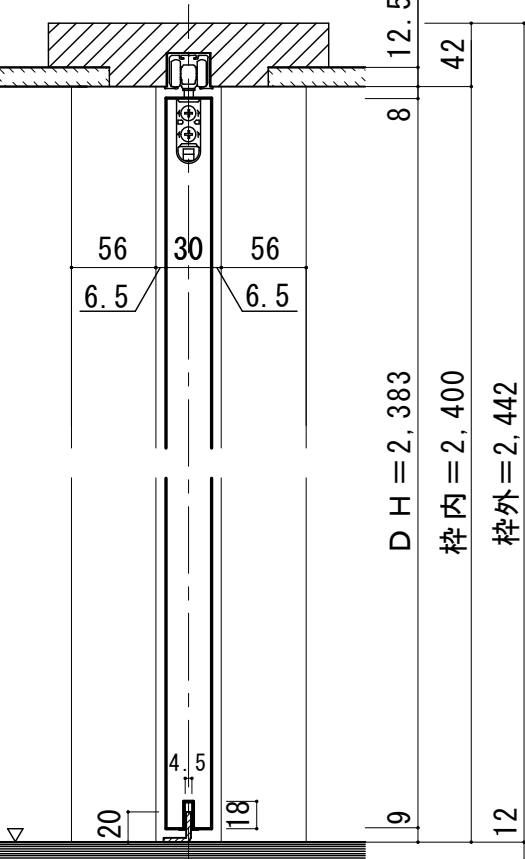
■縦断面図
