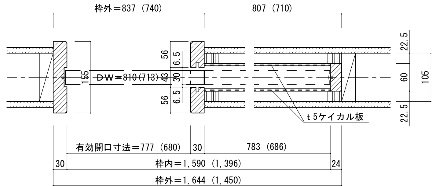
■横断面図
