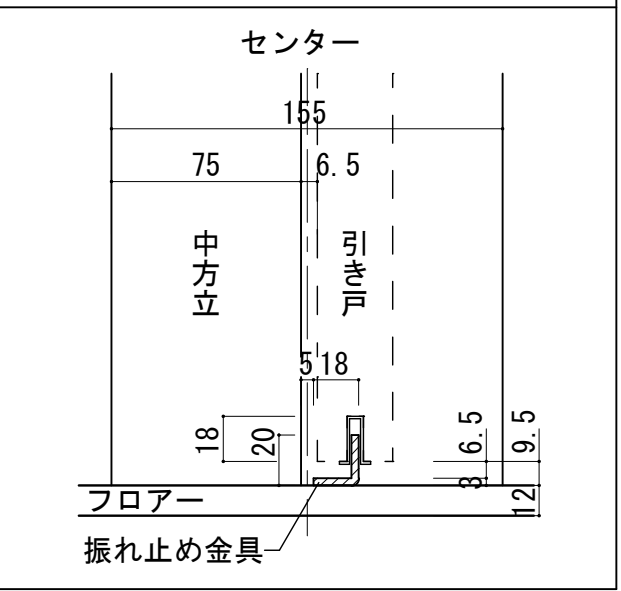
振れ止め金具取り付け位置 S=1/3
