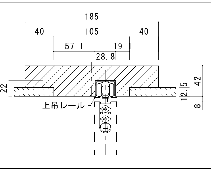
上吊レール取り付け位置 S=1/3
