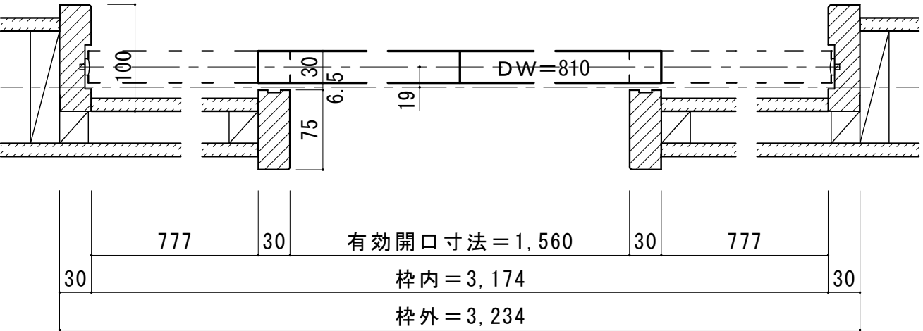
■横断面図
