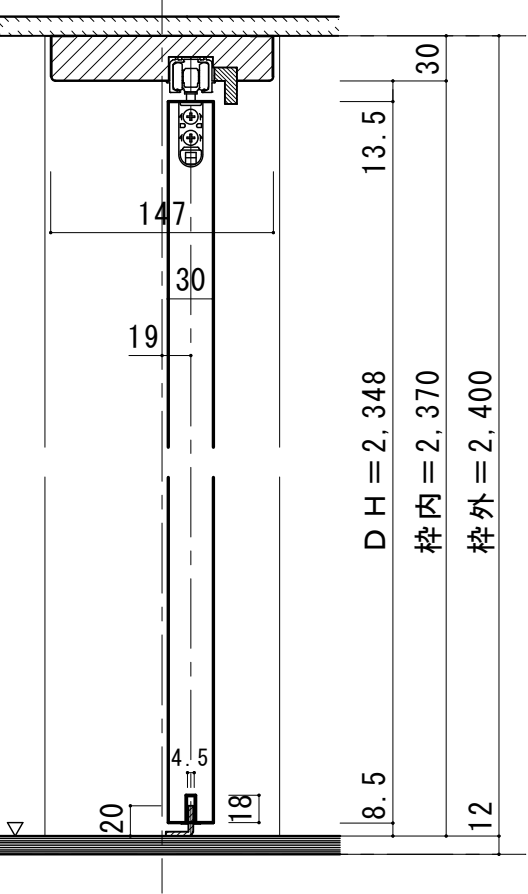
■縦断面図
