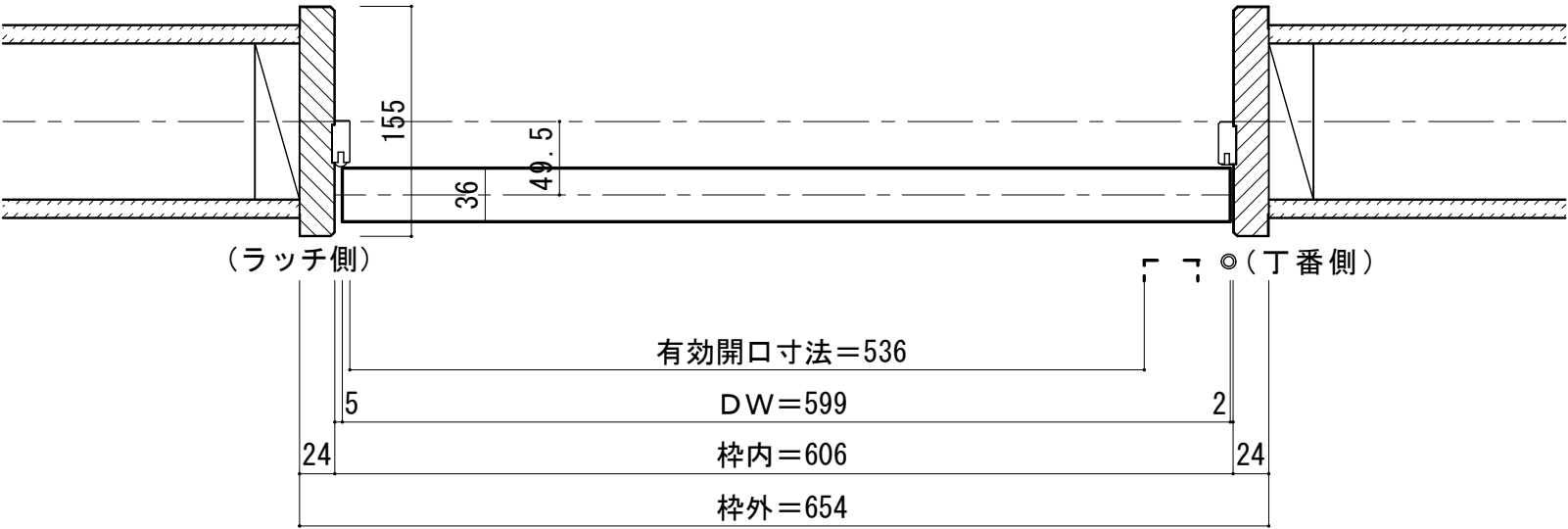
■ 横断面図
