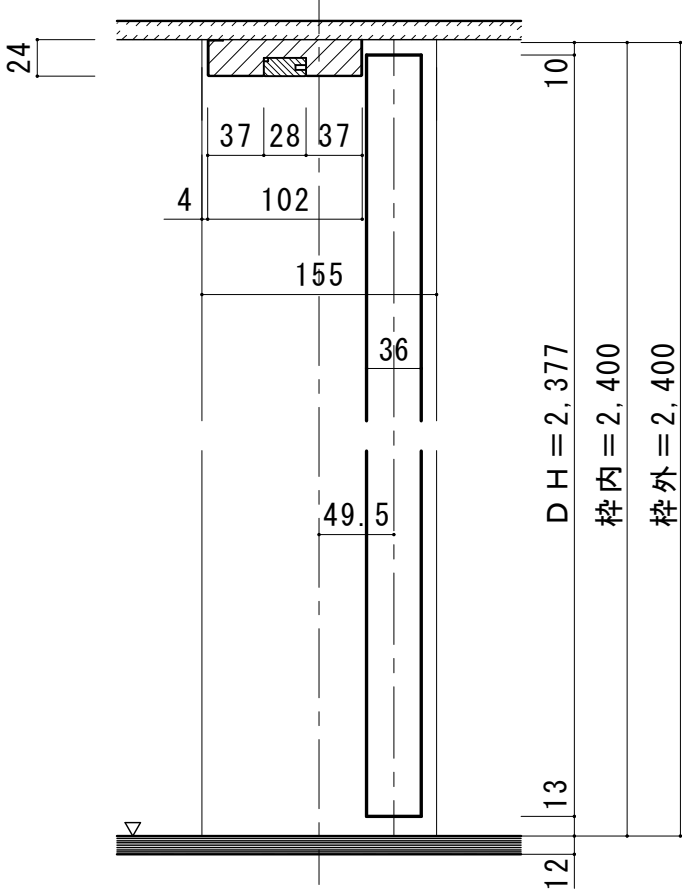
■ 縦断面図
