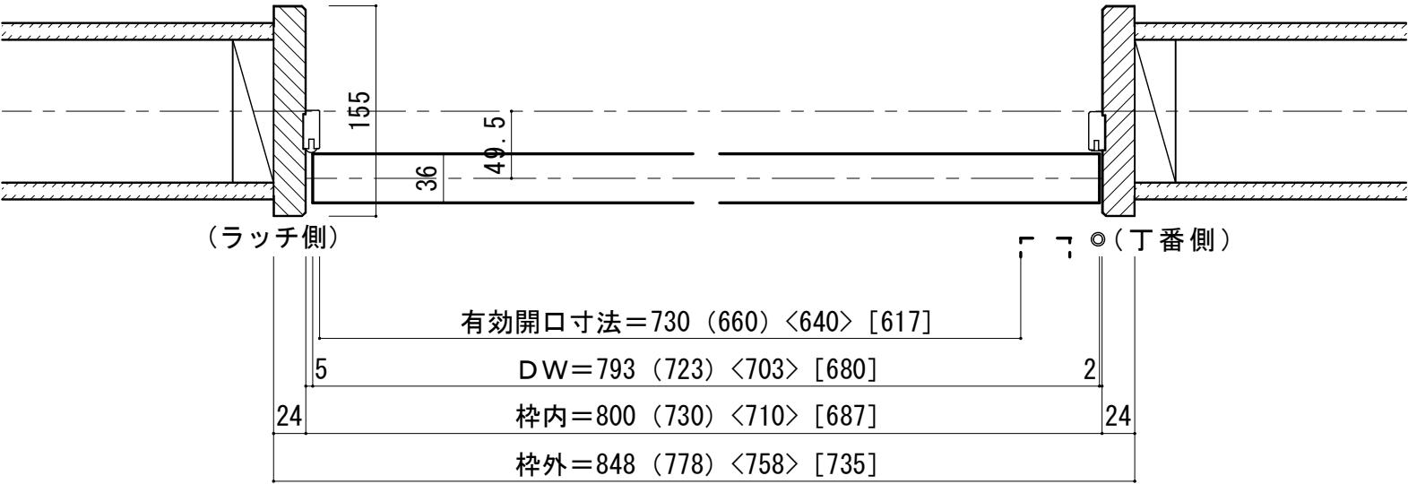
■ 横断面図
