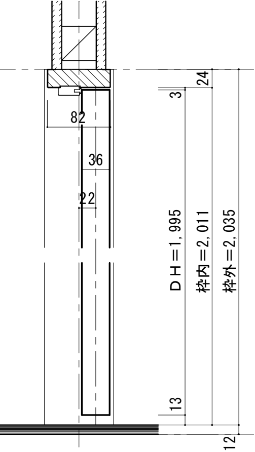
■縦断面図
