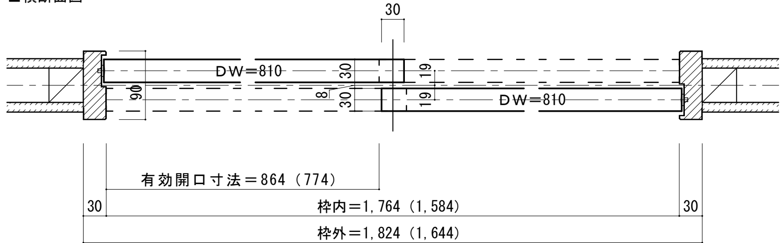
■横断面図
