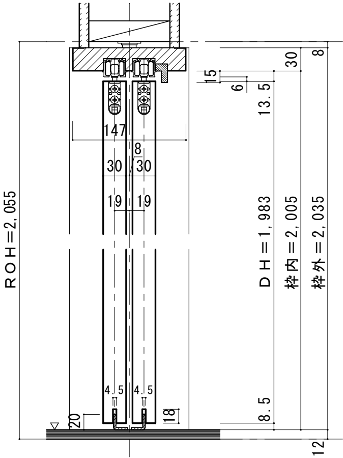
■縦断面図
