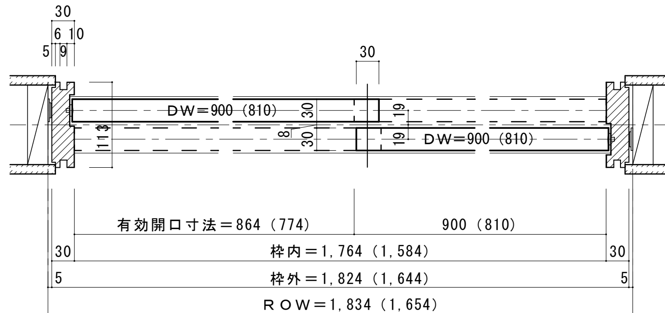
■横断面図
