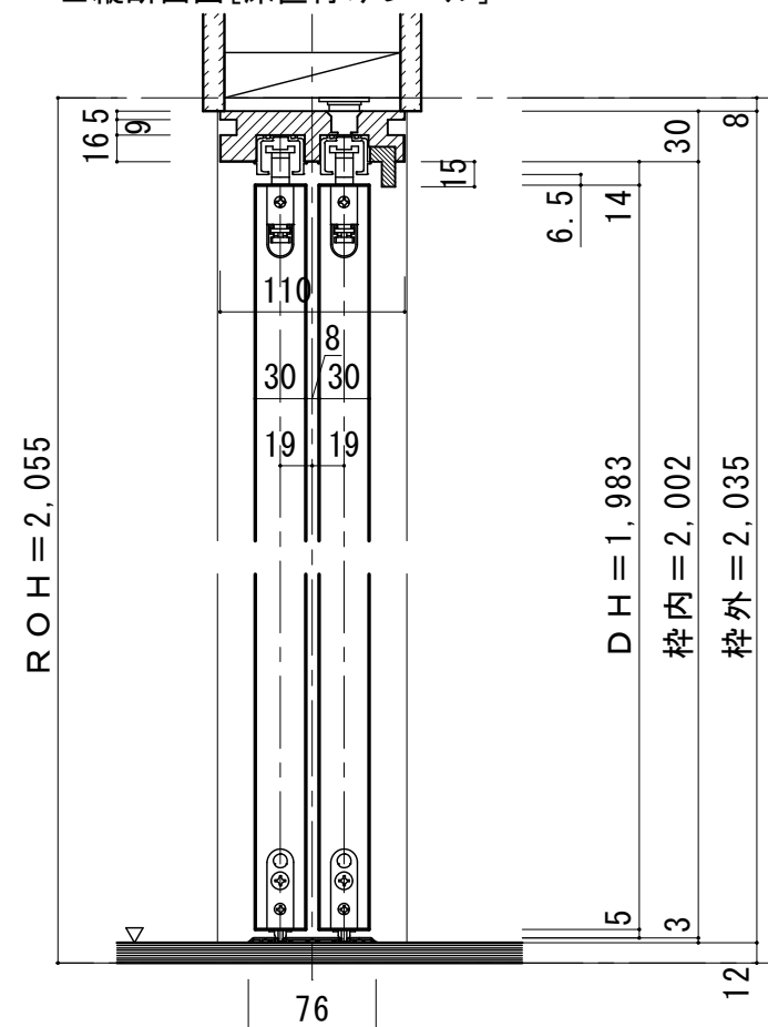
■縦断面図[床直付けレール]
