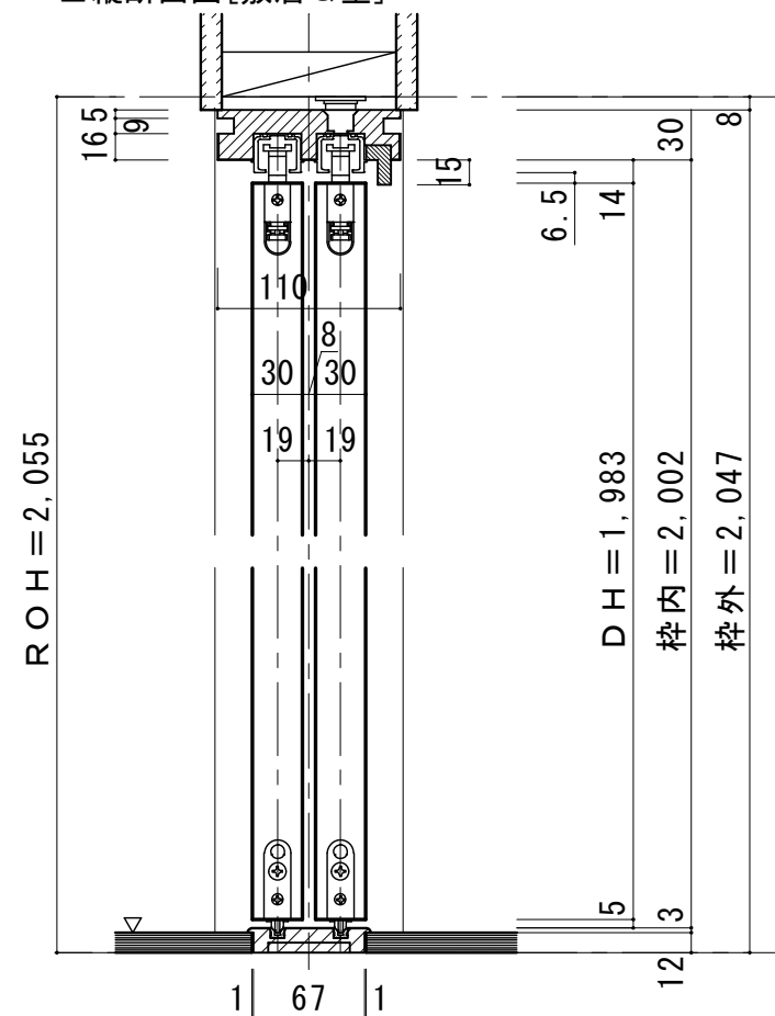
■縦断面図[敷居Q型]
