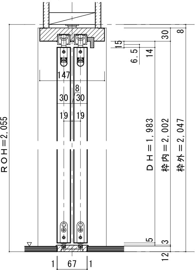
■縦断面図[敷居Q型]
