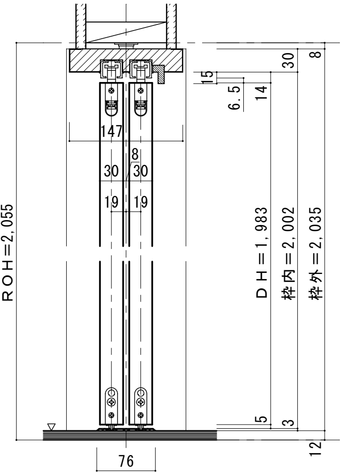
■縦断面図[床直付けレール]
