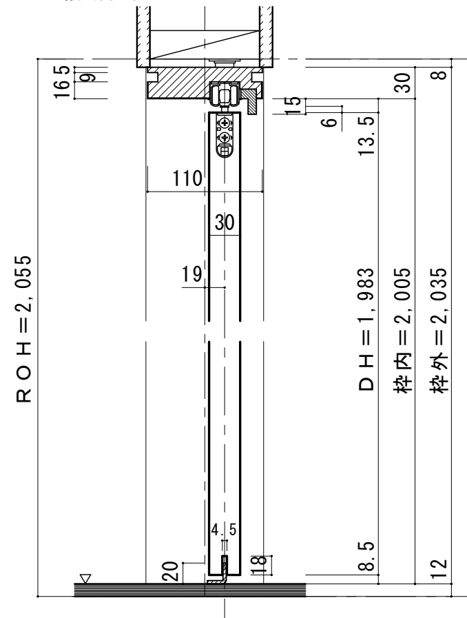
■縦断面図
