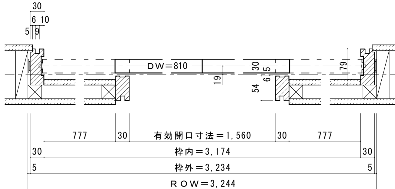
■横断面図
