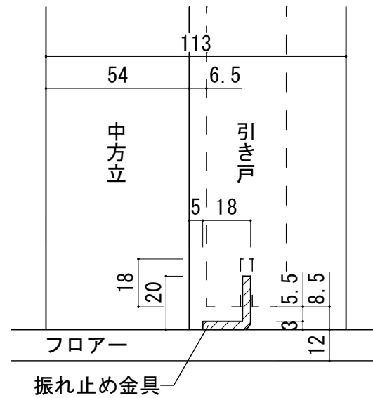
振れ止め金具取り付け位置 (S=1/2)
