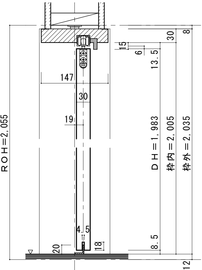
■縦断面図
