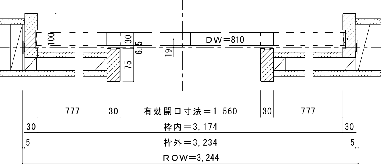
■横断面図
