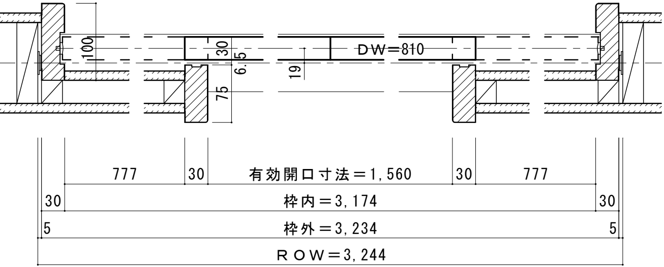
■横断面図
