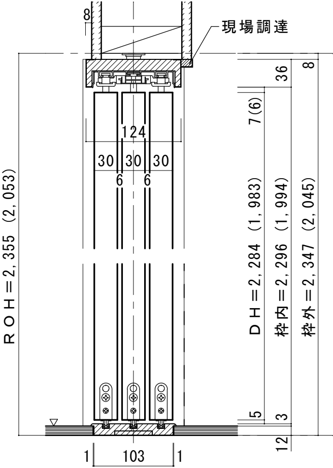
■縦断面図 H=8尺 (H=7尺) [レールタイプ]
